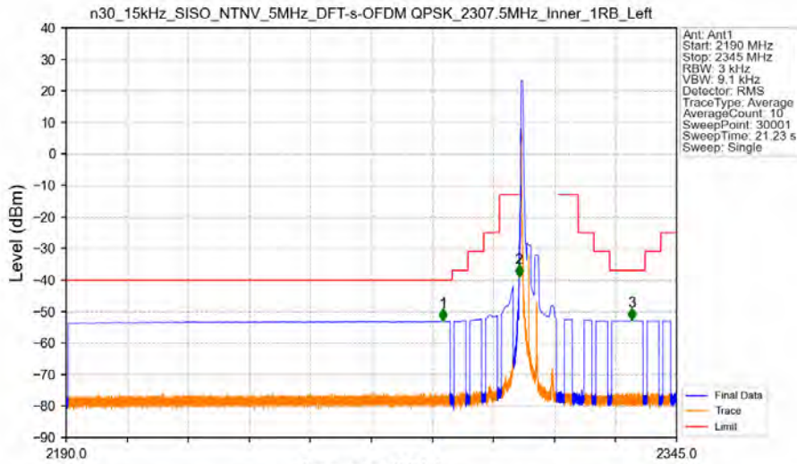
n30_15kHz_SISO_NTNV_5MHz_DFT-s-OFDM QPSK_2307.5MHz_Inner_1RB_Left
