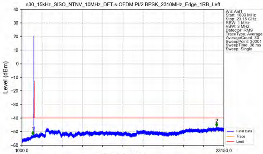
n30_15kHz_SISO_NTNV_10MHz_DFT-s-OFDM PI/2 BPSK_2310MHz_Edge_1RB_Left
