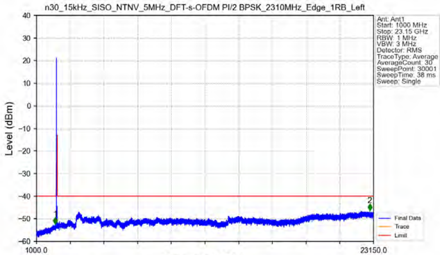
n30_15kHz_SISO_NTNV_5MHz_DFT-s-OFDM PI/2 BPSK_2310MHz_Edge_1RB_Left
