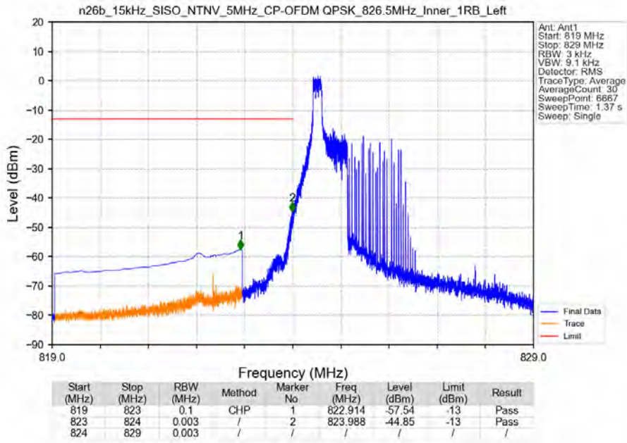
n26b_15kHz_SISO_NTNV_5MHz_CP-OFDM QPSK_826.5MHz_Inner_1RB_Left
