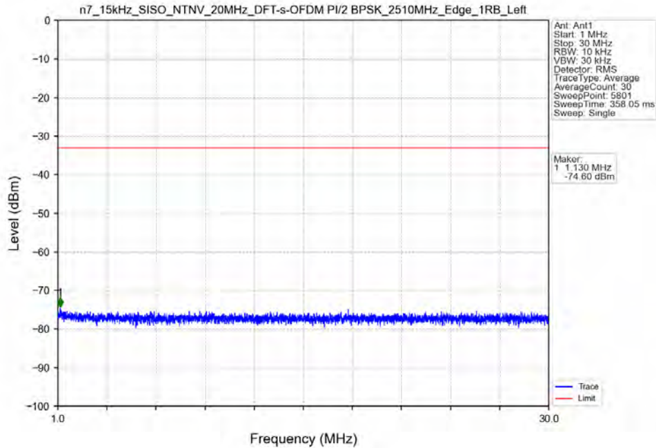
n7_15kHz_SISO_NTNV_20MHz_DFT-s-OFDM PI/2 BPSK_2510MHz_Edge_1RB_Left
