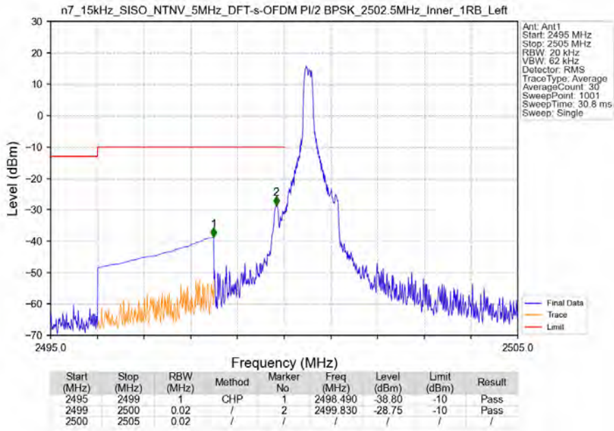
n7_15kHz_SISO_NTNV_5MHz_DFT-s-OFDM PI/2 BPSK_2502.5MHz_Inner_1RB_Left
