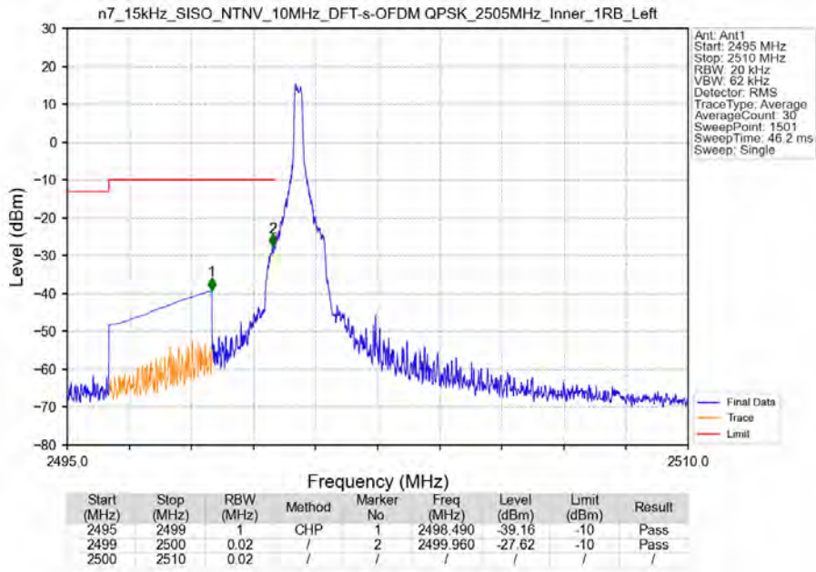
n7_15kHz_SISO_NTNV_10MHz_DFT-s-OFDM QPSK_2505MHz_Inner_1RB_Left
