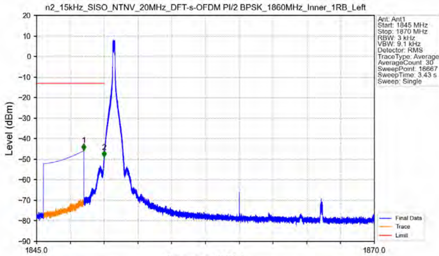
n2_15kHz_SISO_NTNV_20MHz_DFT-s-OFDM PI/2 BPSK_1860MHz_Inner_1RB_Left
