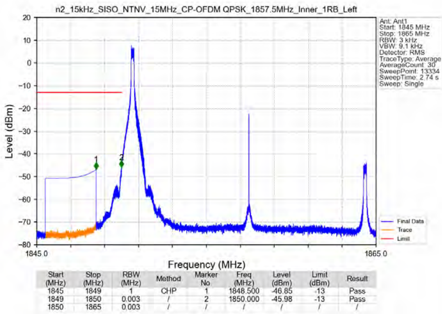
n2_15kHz_SISO_NTNV_15MHz_CP-OFDM QPSK_1857.5MHz_Inner_1RB_Left
