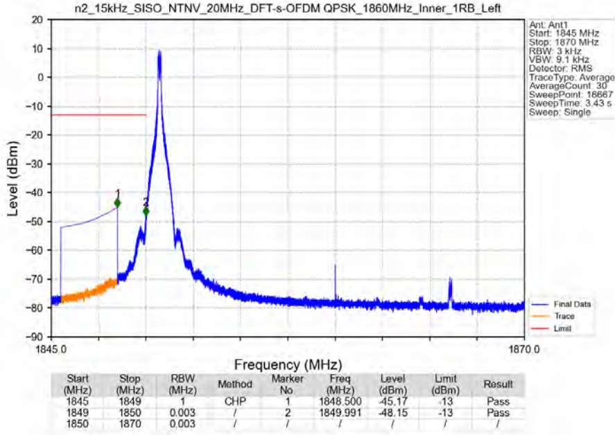
n2_15kHz_SISO_NTNV_20MHz_DFT-s-OFDM QPSK_1860MHz_Inner_1RB_Left
