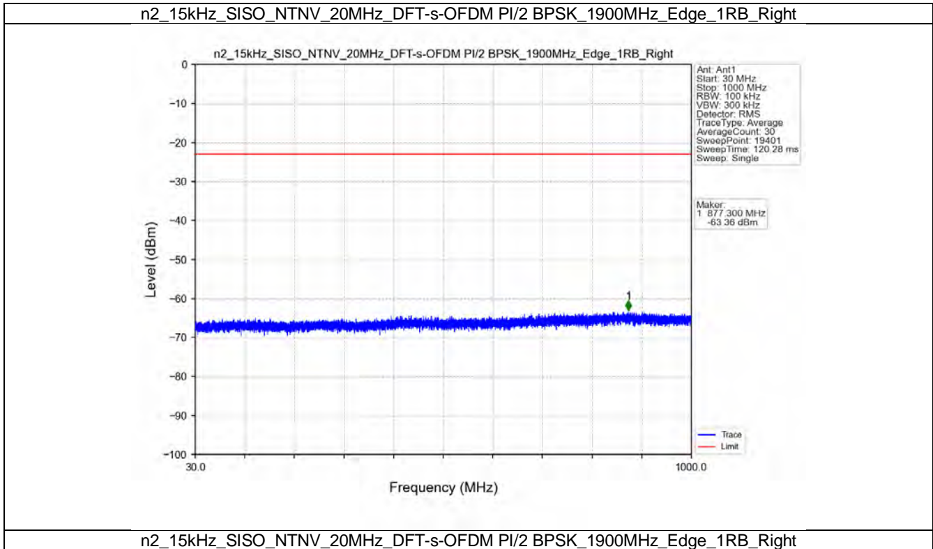
n2_15kHz_SISO_NTNV_20MHz_DFT-s-OFDM PI/2 BPSK_1900MHz_Edge_1RB_Right
