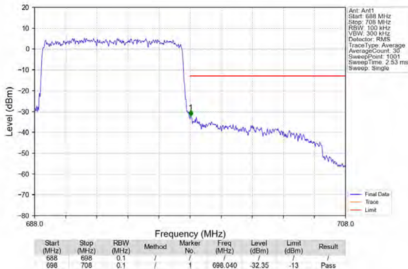
Band71 10MHz QPSK HCH 693MHz RB 50_0 NTV
