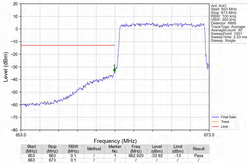
Band71_10MHz_QPSK_LCH_668MHz_RB_50_0_NTNV
