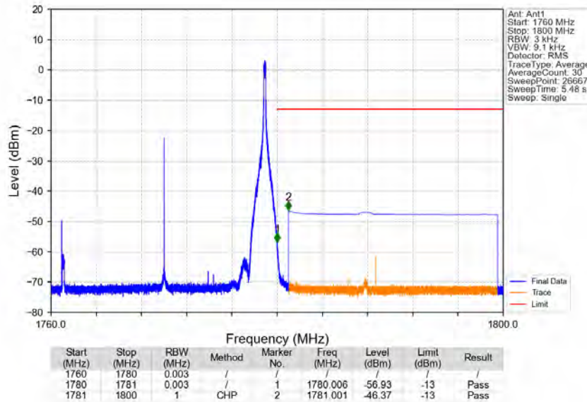
Band66_20MHz_256QAM_HCH_1770MHz_RB_1_99_NTNV
