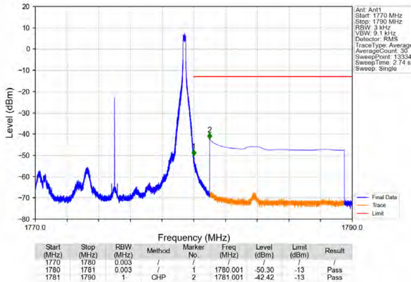
Band66_10MHz_QPSK_HCH_1775MHz_RB_1_49_NTNV
