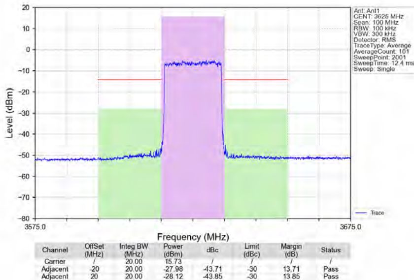
Band48 20MHz 256QAM MCH 3625MHz RB 100 0 NTN
