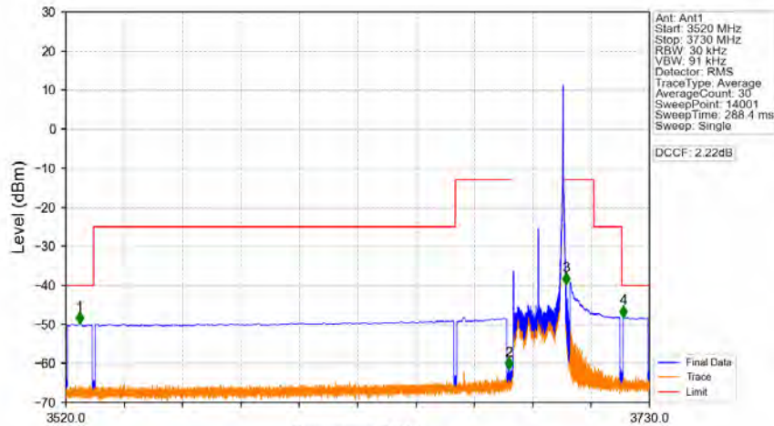
Band48_20MHz_256QAM_HCH_3690MHz_RB_1_99_NTNV
