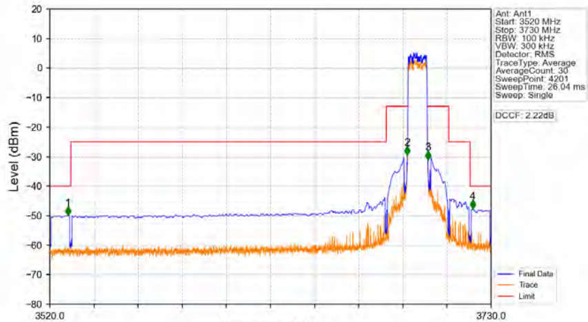
Band48_10MHz_QPSK_HCH_3695MHz_RB_50_0_NTNV
