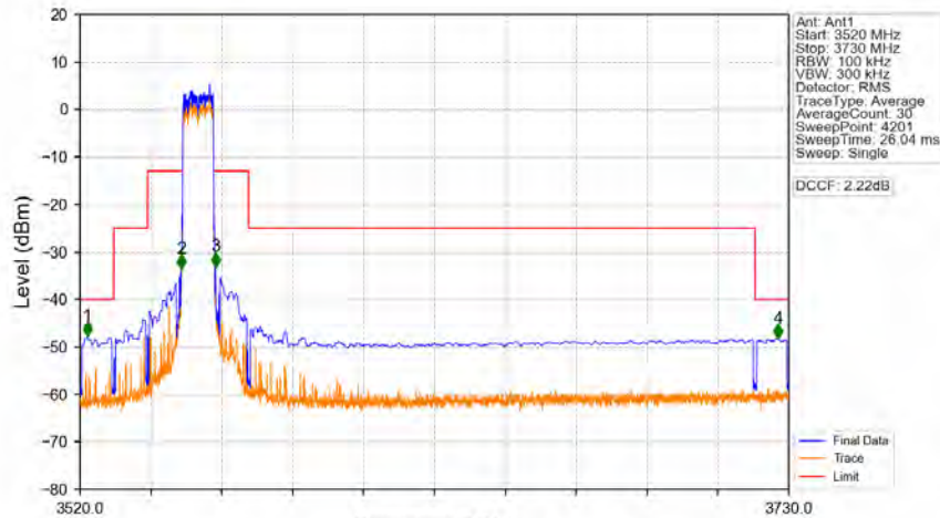
Band48_10MHz_QPSK_LCH_3555MHz_RB_50_0_NTNV
