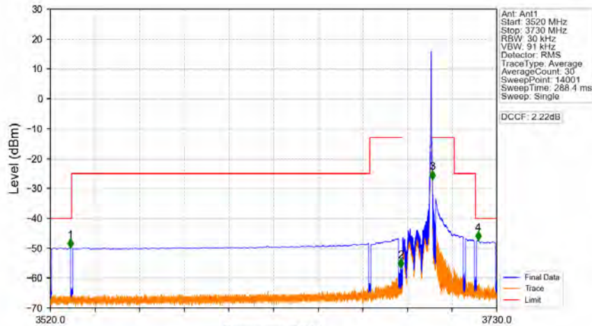
Band48_15MHz_16QAM_HCH_3692.5MHz_RB_1_74_NTNV
