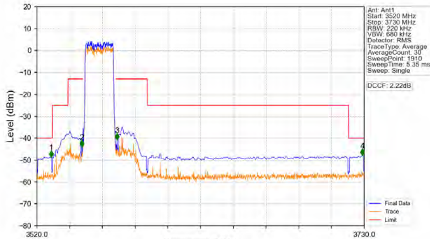
Band48 20MHz QPSK LCH 3560MHz RB 100 0 NTN
