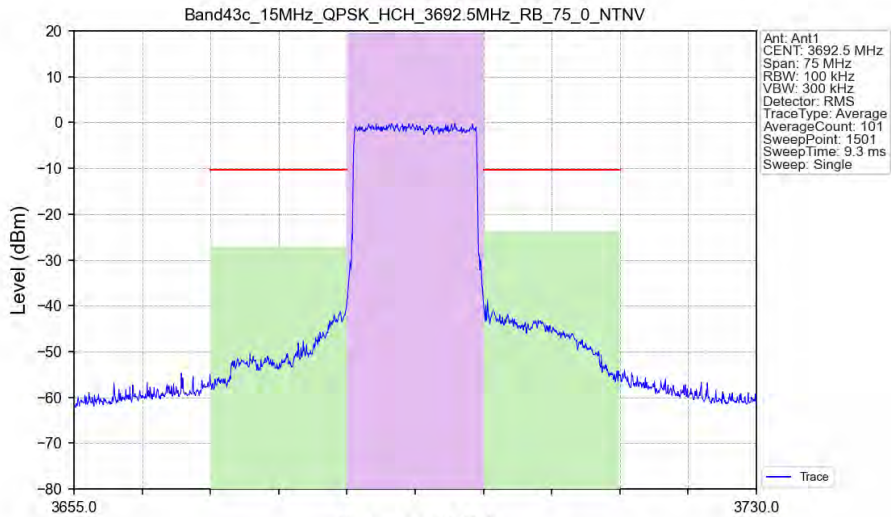
Band43c_15MHz_QPSK_HCH_3692.5MHz_RB_75_0_NTNV
