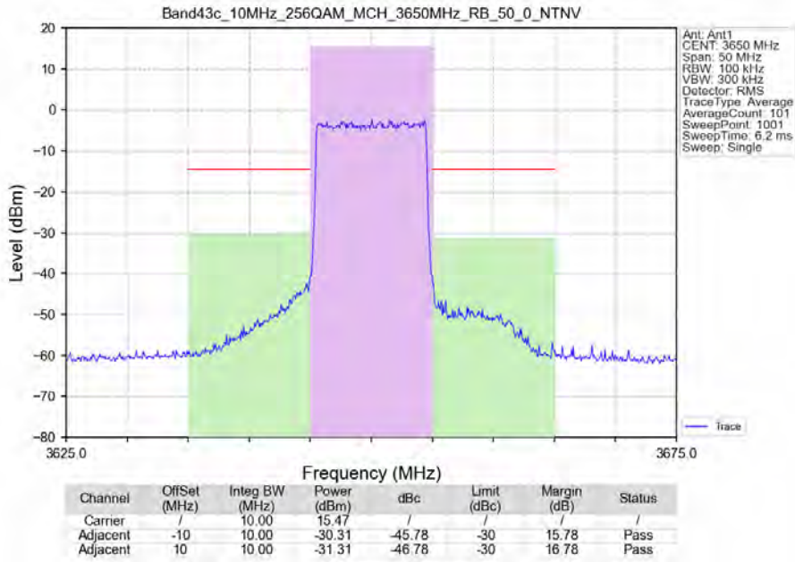
Band43c_10MHz_256QAM_MCH_3650MHz_RB_50_0_NTNV
