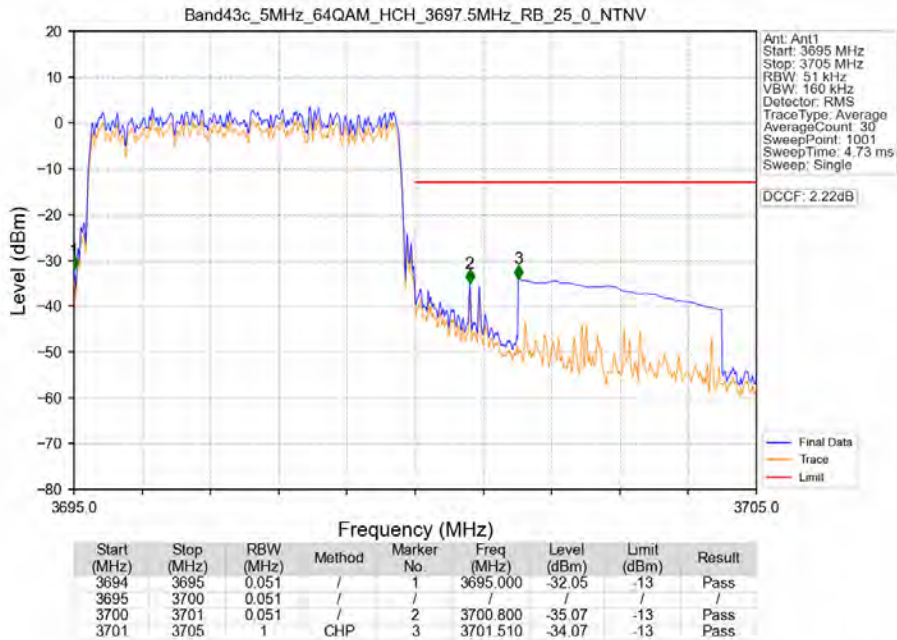
Band43c 5MHz 64QAM HCH 3697.5MHz RB 25 0 NTV
