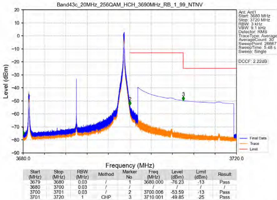
Band43c_20MHz_256QAM_HCH_3690MHz_RB_1_99_NTNV
