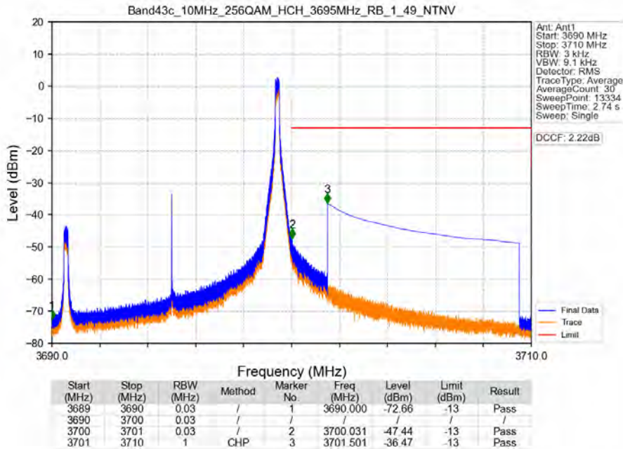
Band43c_10MHz_256QAM_HCH_3695MHz_RB_1_49_NTNV
