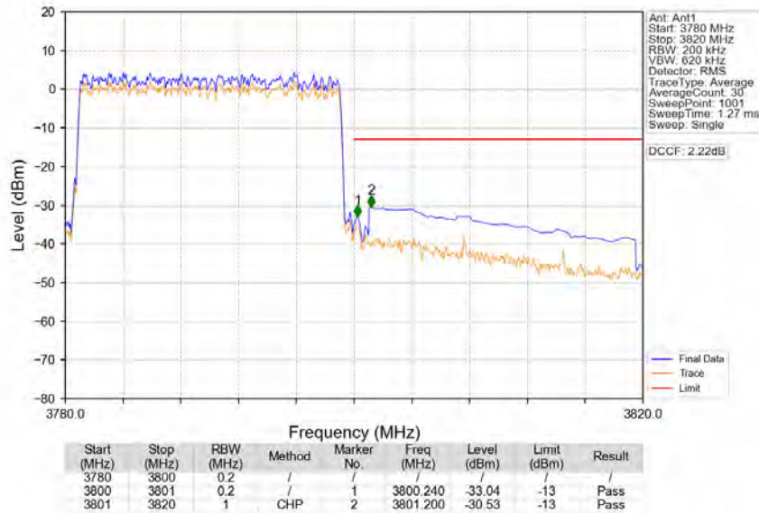
Band43d_20MHz_QPSK_HCH_3790MHz_RB_100_0_NTNV
