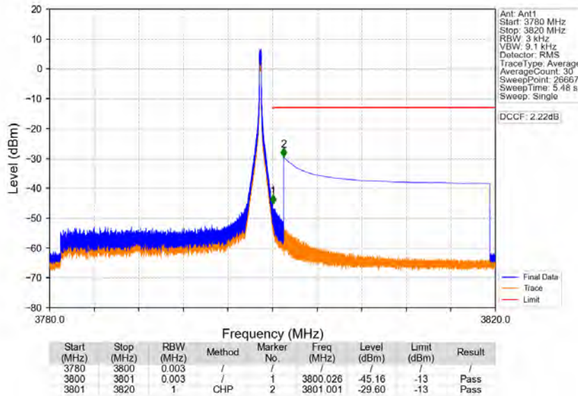
Band43d_20MHz_16QAM_HCH_3790MHz_RB_1_99_NTNV
