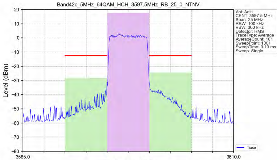
Band42c 5MHz 64QAM HCH 3597.5MHz RB 25 0 NTV
