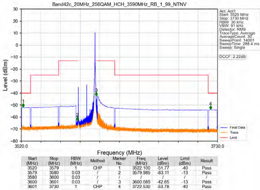
Band42c_20MHz_256QAM_HCH_3590MHz_RB_1_99_NTNV
