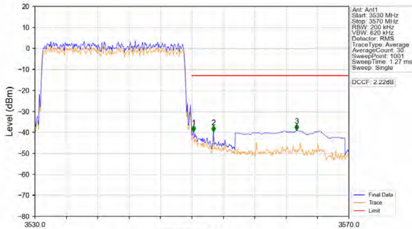
Band42a_20MHz_QPSK_HCH_3540MHz_RB_100_0_NTNV
