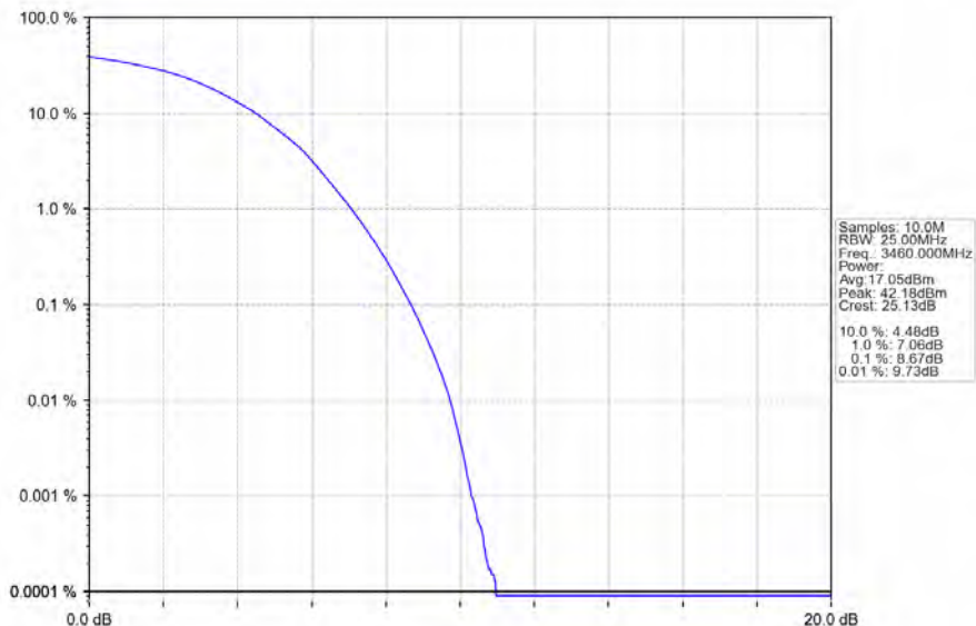
Band42a 20MHz 64QAM LCH 3460MHz RB 100 0 NTN
