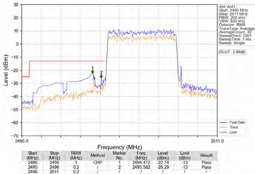
Band41_10MHz_QPSK_LCH_2501MHz_RB_50_0_NTNV
