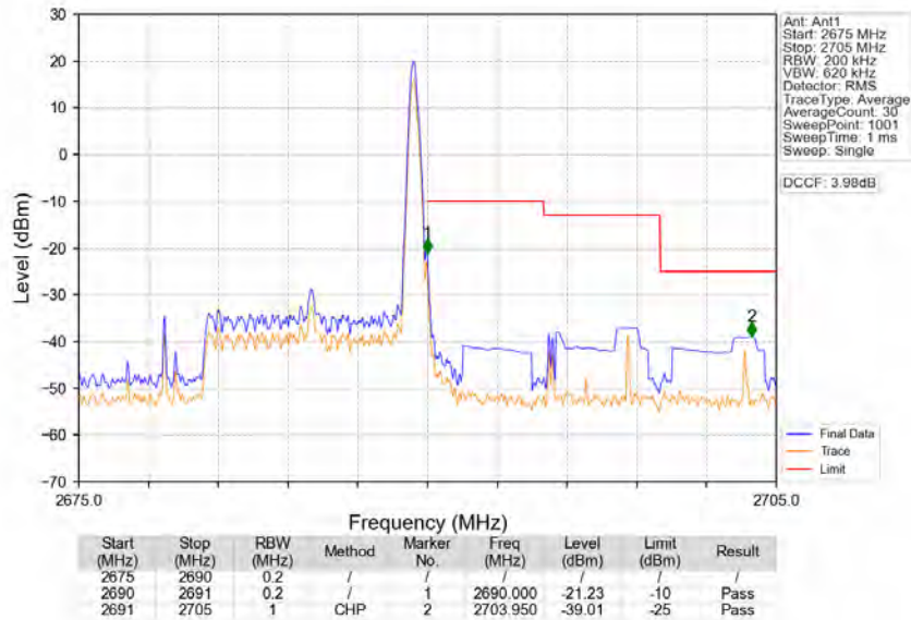
Band41_10MHz_256QAM_HCH_2685MHz_RB_1_49_NTNV
