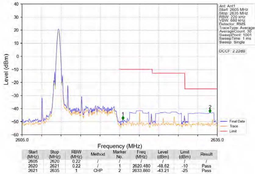
Band38_10MHz_QPSK_HCH_2615MHz_RB_50_0_NTNV
