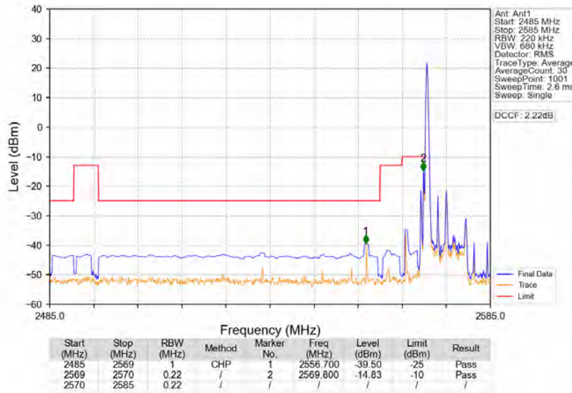
Band38_10MHz_QPSK_LCH_2575MHz_RB_50_0_NTNV
