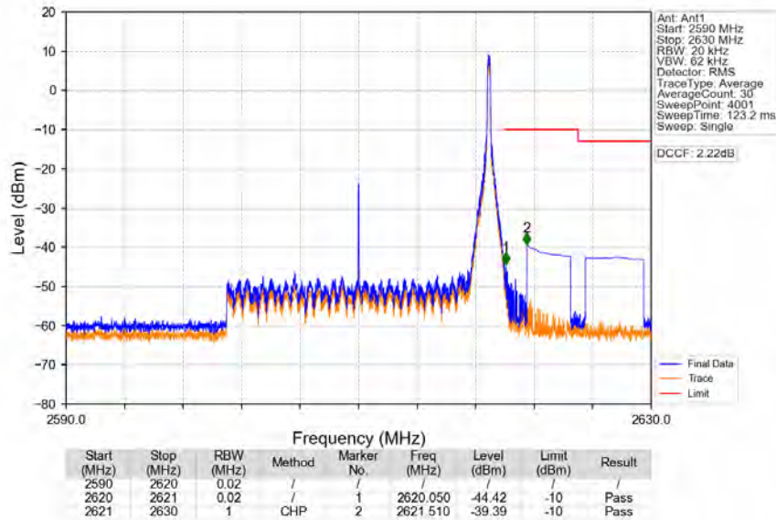
Band38_20MHz_256QAM_HCH_2610MHz_RB_1_99_NTNV
