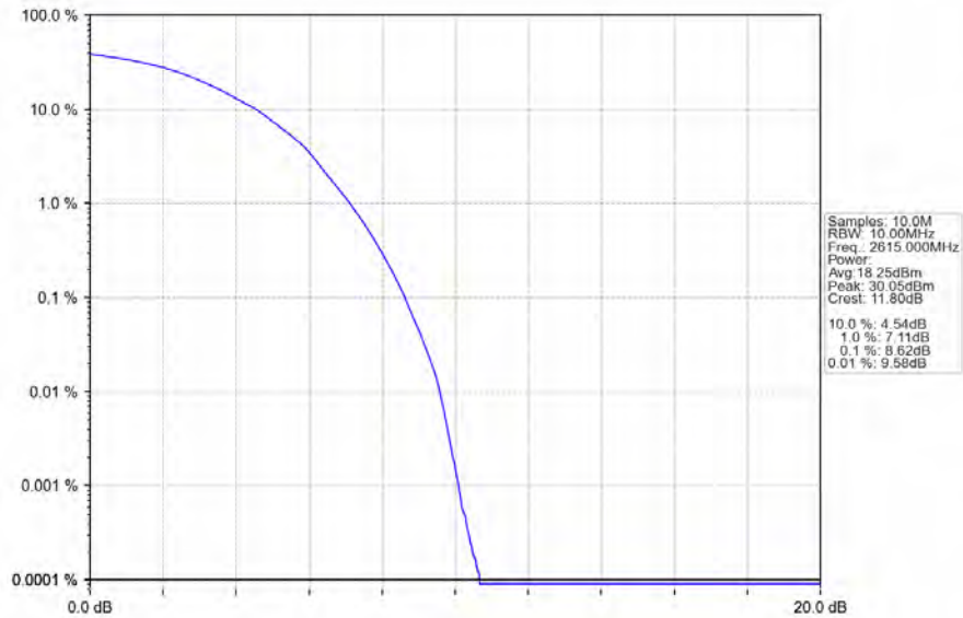
Band38_10MHz_QPSK_HCH_2615MHz_RB_50_0_NTNV
