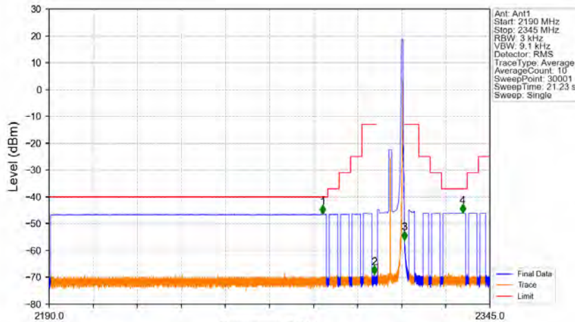
Band30_10MHz_256QAM_MCH_2310MHz_RB_1_49_NTNV
