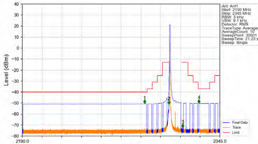
Band30_10MHz_QPSK_MCH_2310MHz_RB_1_0_NTNV
