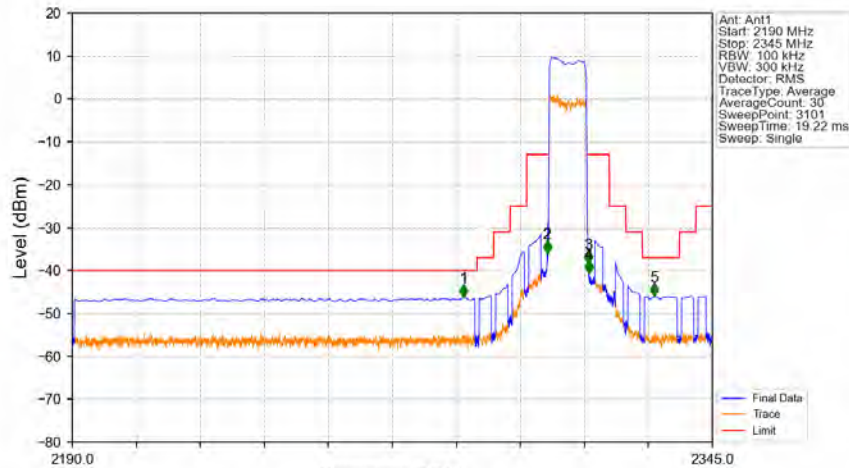
Band30_10MHz_256QAM_LCH_2310MHz_RB_50_0_NTNV
