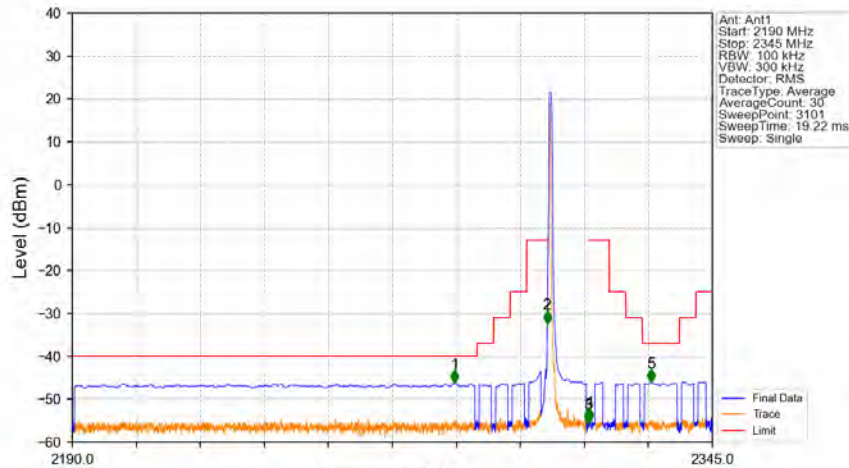
Band30_10MHz_QPSK_HCH_2310MHz_RB_50_0_NTNV
