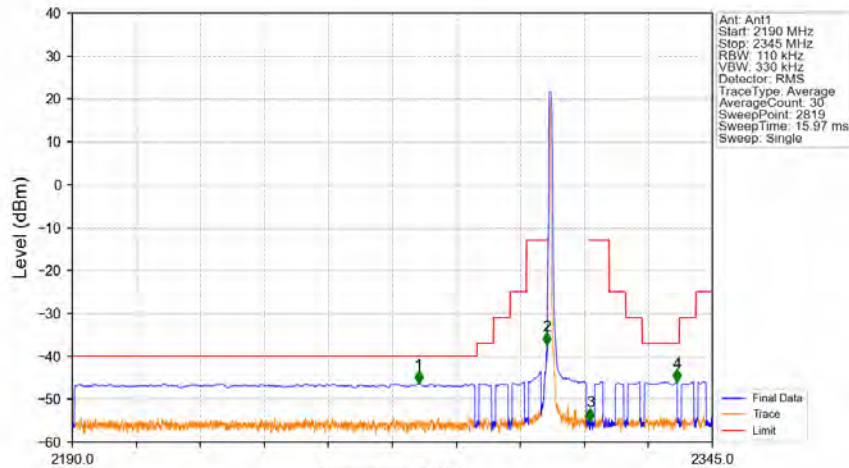
Band30_10MHz_QPSK_MCH_2310MHz_RB_50_0_NTNV
