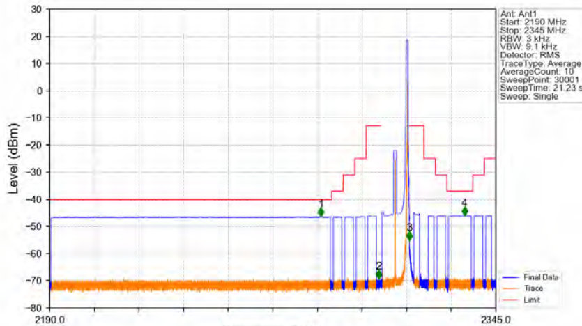
Band30_10MHz_256QAM_HCH_2310MHz_RB_1_49_NTNV
