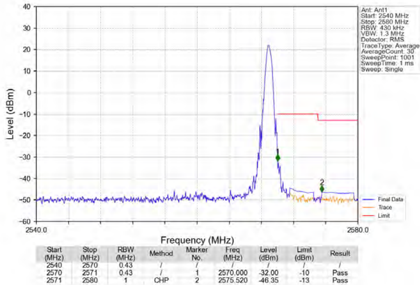
Band7_20MHz_16QAM_HCH_2560MHz_RB_1_99_NTNV
