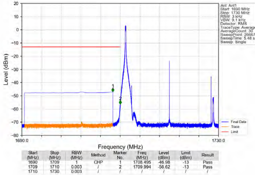
Band4_20MHz_256QAM_LCH_1720MHz_RB_1_0_NTNV
