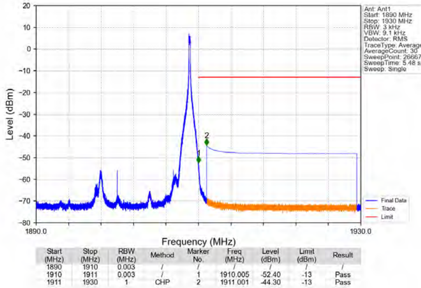
Band2_20MHz_QPSK_HCH_1900MHz_RB_1_99_NTNV
