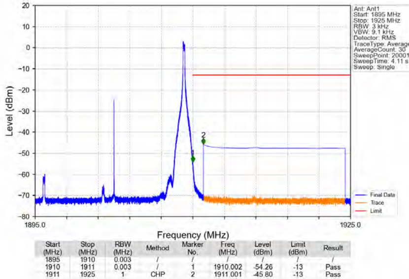
Band2_15MHz_256QAM_HCH_1902.5MHz_RB_1_74_NTNV
