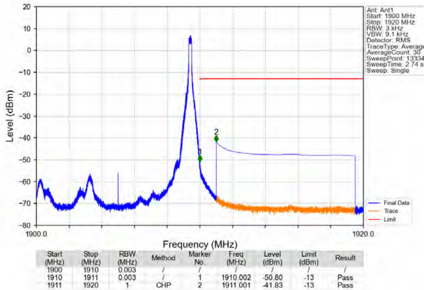
Band2_10MHz_QPSK_HCH_1905MHz_RB_1_49_NTNV
