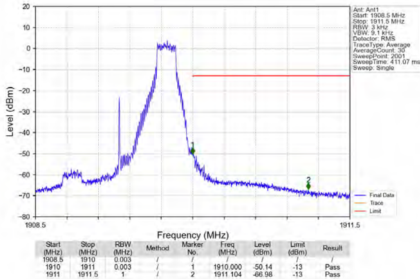
Band2 1.4MHz 256QAM HCH 1909.3MHz RB 1 5 NTV
