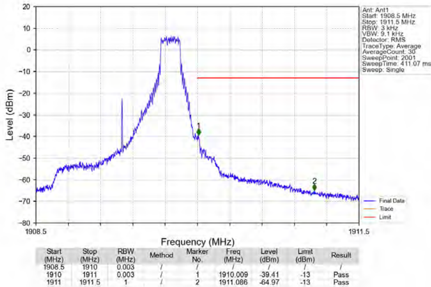
Band2 1.4MHz QPSK HCH 1909.3MHz RB 1 5 NTV
