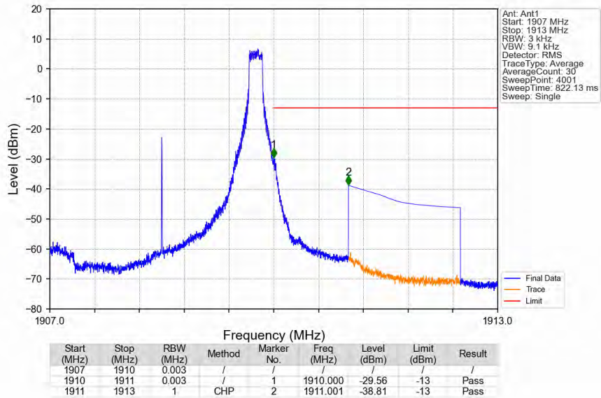
Band2_3MHz_QPSK_HCH_1908.5MHz_RB_1_14_NTNV
