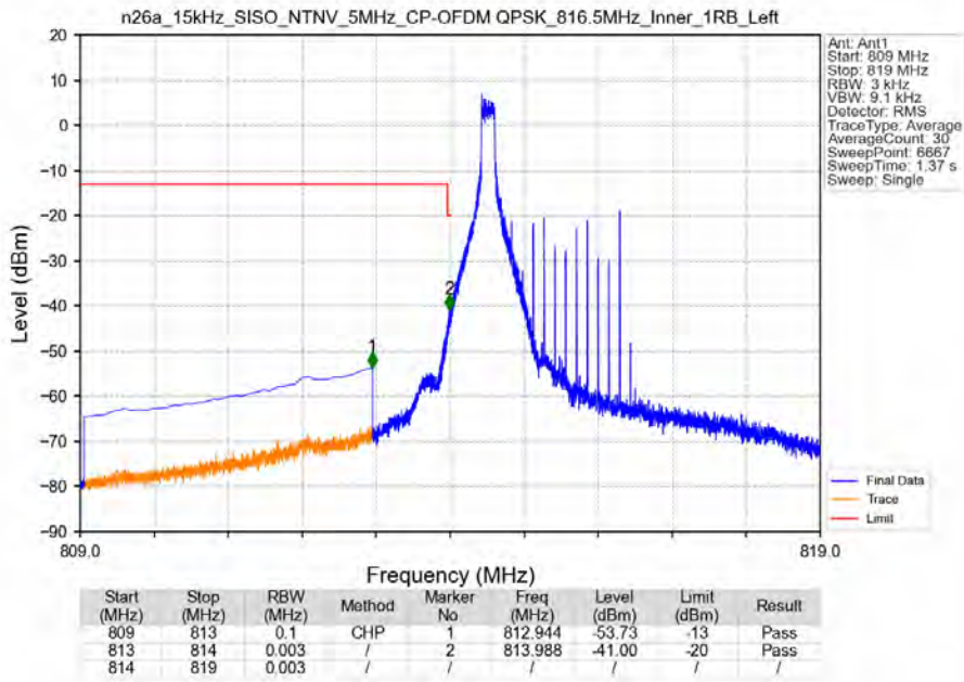
n26a_15kHz_SISO_NTNV_5MHz_CP-OFDM QPSK_816.5MHz_Inner_1RB_Left
