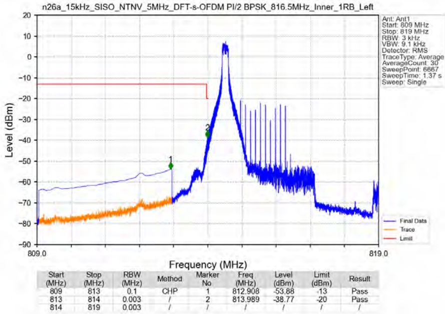
n26a_15kHz_SISO_NTNV_5MHz_DFT-s-OFDM PI/2 BPSK_816.5MHz_Inner_1RB_Left
