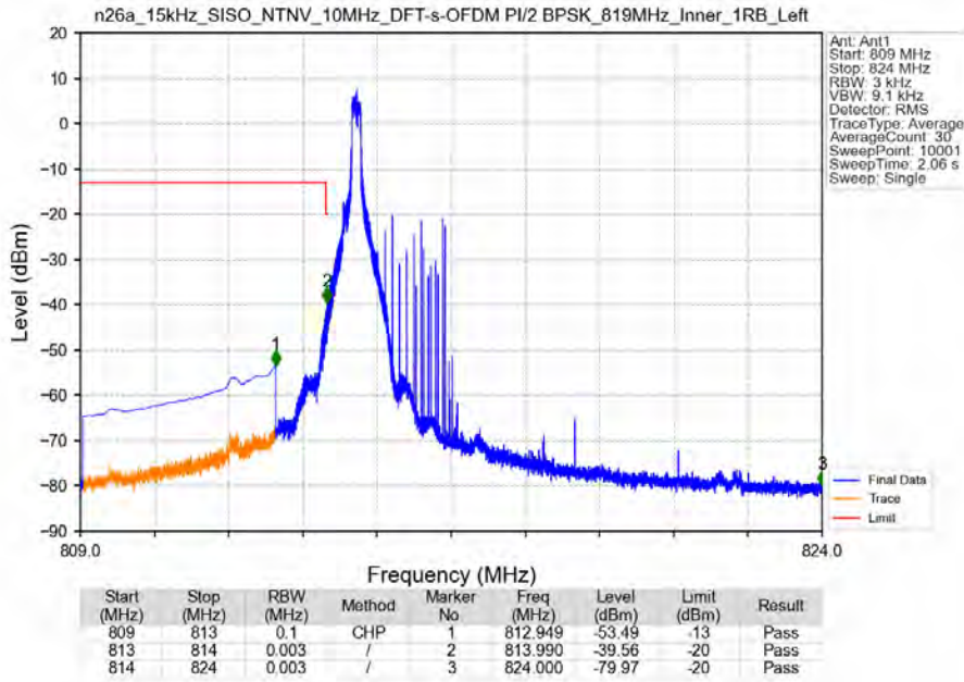
n26a_15kHz_SISO_NTNV_10MHz_DFT-s-OFDM PI/2 BPSK_819MHz_Inner_1RB_Left
