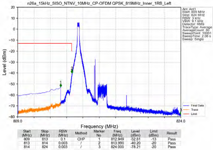
n26a_15kHz_SISO_NTNV_10MHz_CP-OFDM QPSK_819MHz_Inner_1RB_Left
