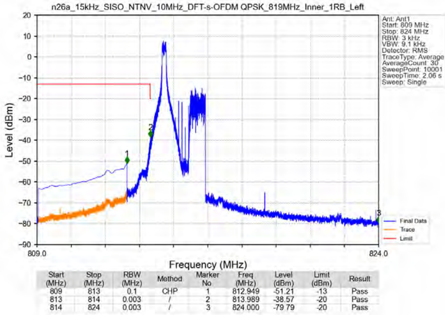
n26a_15kHz_SISO_NTNV_10MHz_DFT-s-OFDM QPSK_819MHz_Inner_1RB_Left
