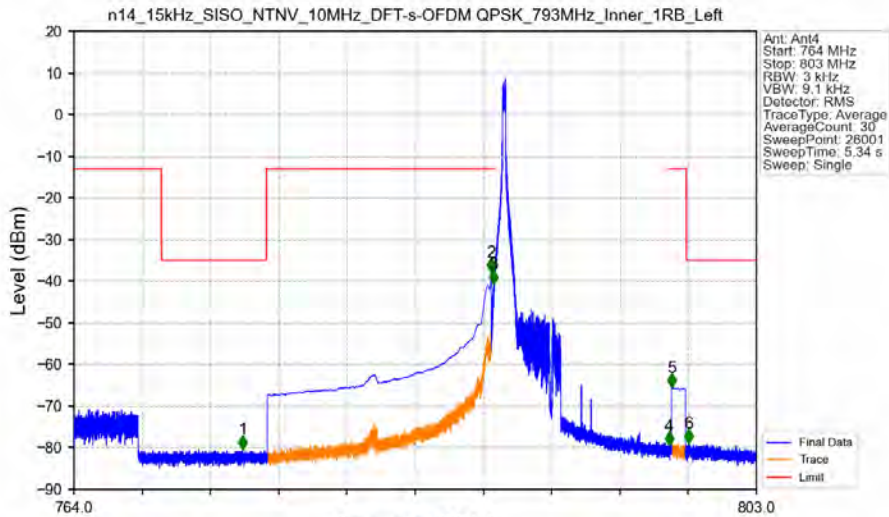
n14_15kHz_SISO_NTNV_10MHz_DFT-s-OFDM QPSK_793MHz_Inner_1RB_Left
