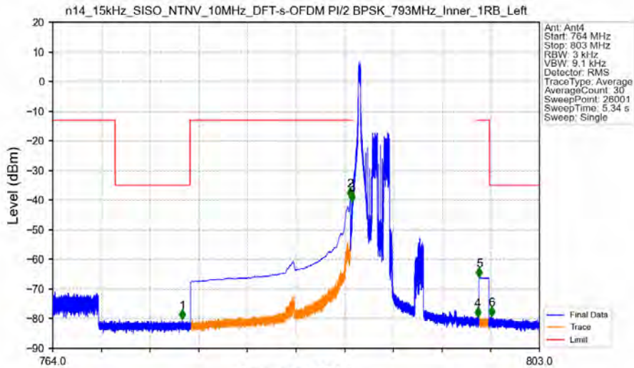
n14_15kHz_SISO_NTNV_10MHz_DFT-s-OFDM PI/2 BPSK_793MHz_Inner_1RB_Left
