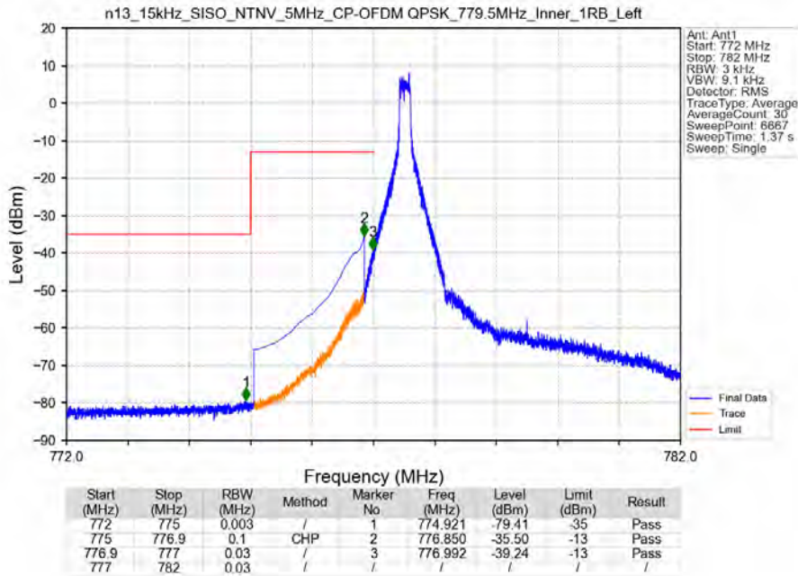
n13_15kHz_SISO_NTNV_5MHz_CP-OFDM_QPSK_779.5MHz_Inner_1RB_Left
