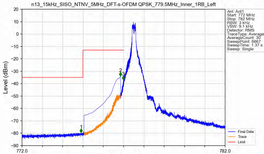
n13_15kHz_SISO_NTNV_5MHz_DFT-s-OFDM_QPSK_779.5MHz_Inner_1RB_Left
