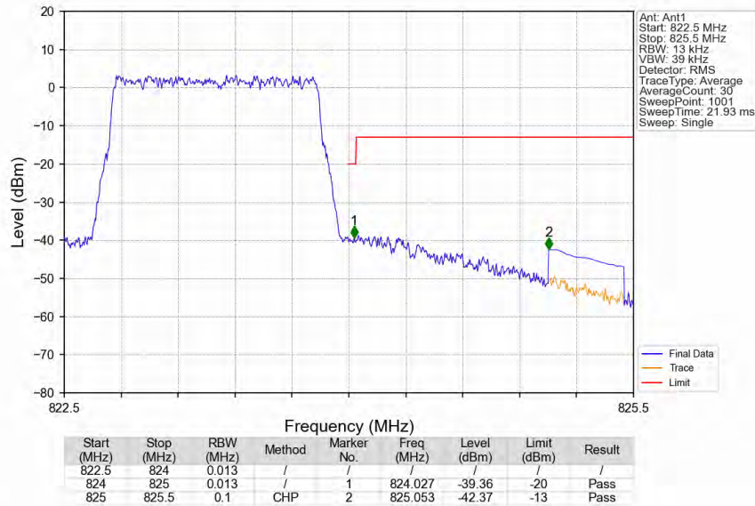
Band26a 1.4MHz 64QAM HCH 823.3MHz RB 6 0 NTV
