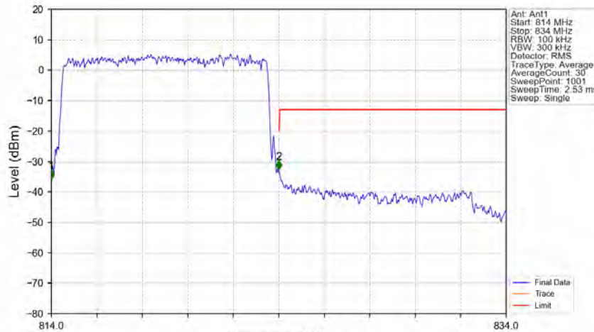
Band26a_10MHz_QPSK_MCH_819MHz_RB_50_0_NTNV
