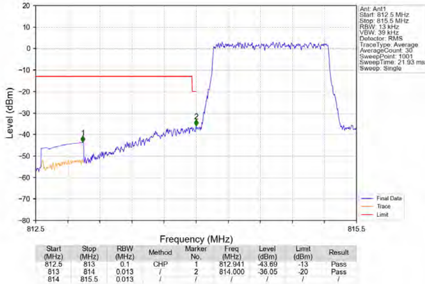
Band26a 1.4MHz 64QAM LCH 814.7MHz RB 6 0 NTV
