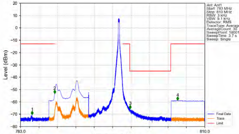
Band14 10MHz QPSK HCH 793MHz RB 1 49 NTNV
