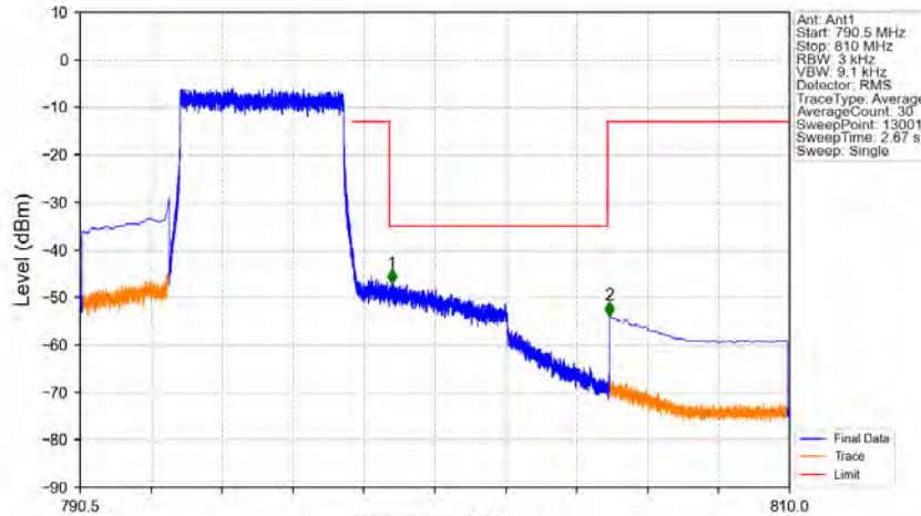
Band14 5MHz QPSK HCH 795.5MHz RB 25 0 NTV
