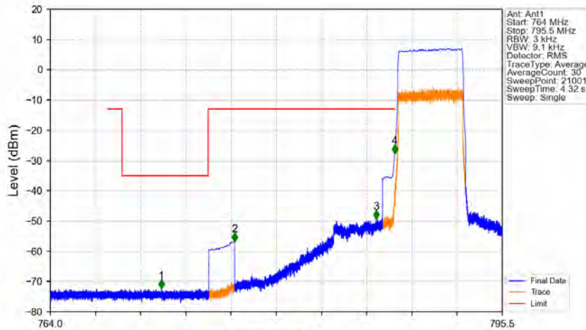
Band14 5MHz QPSK LCH 790.5MHz RB 25 0 NTVV
