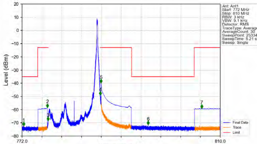
Band13 10MHz QPSK HCH 782MHz RB 1 49 NTNV
