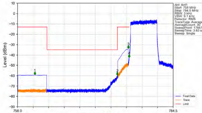
Band13 5MHz QPSK LCH 779.5MHz RB 25 0 NTV
