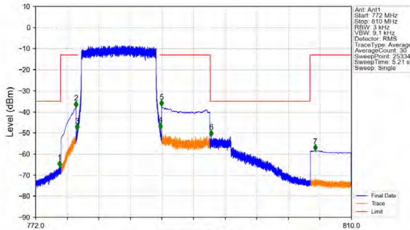
Band13 10MHz QPSK MCH 782MHz RB 50 0 NTN
