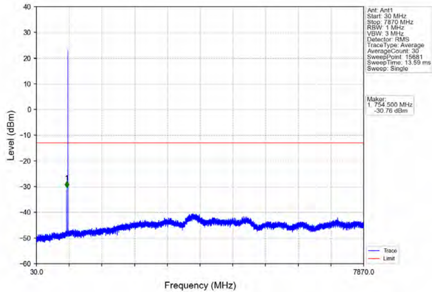
Band13 5MHz QPSK HCH 784.5MHz RB 1 0 NTV
