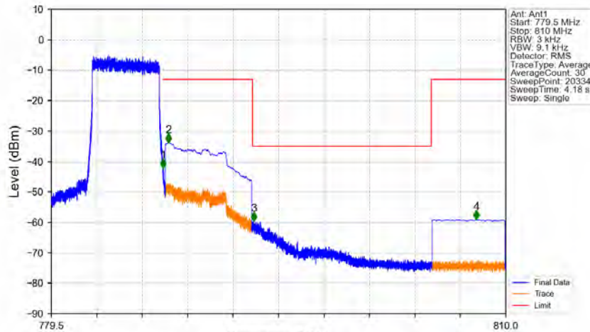
Band13 5MHz QPSK HCH 784.5MHz RB 25 0 NTV
