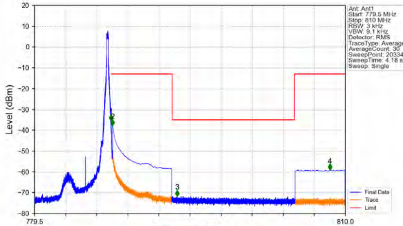
Band13 5MHz 16QAM HCH 784.5MHz RB 1 24 NTNV
