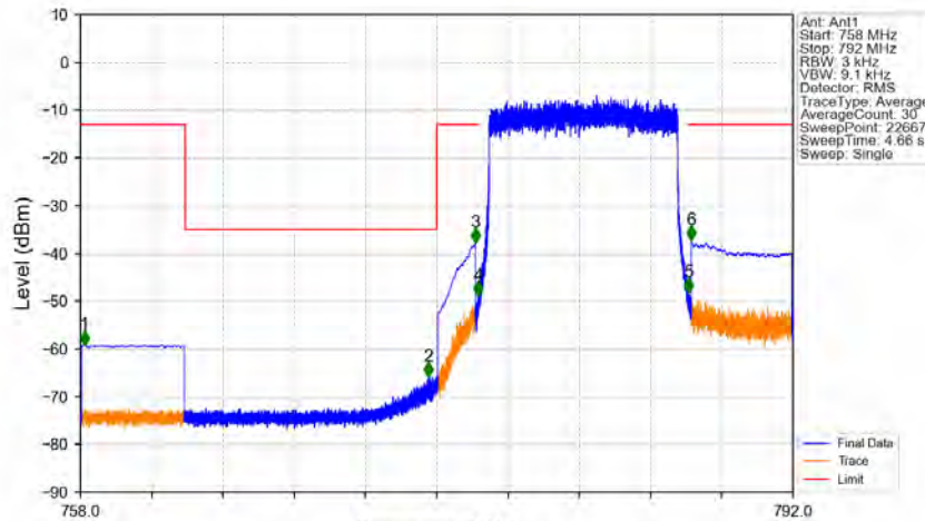
Band13 10MHz QPSK LCH 782MHz RB 50 0 NTN
