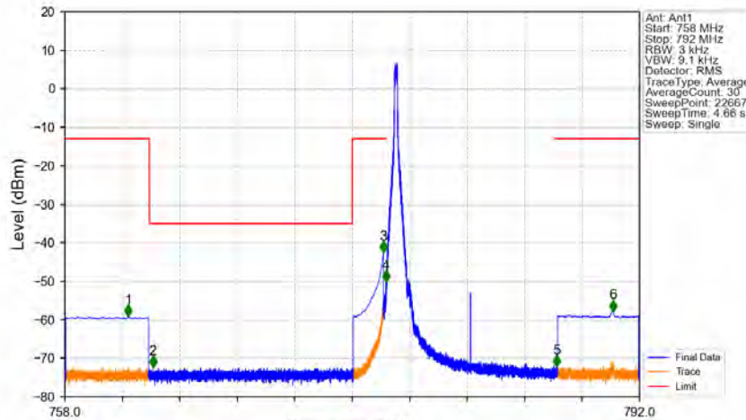
Band13 10MHz 64QAM LCH 782MHz RB 1 0 NTN
