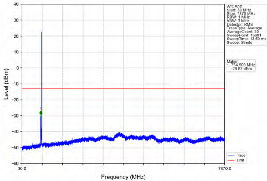
Band13 10MHz QPSK MCH 782MHz RB 1 0 NTNV
