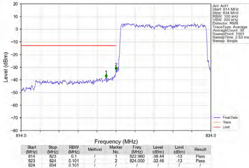
Band5_10MHz_QPSK_LCH_829MHz_RB_50_0_NTNV
