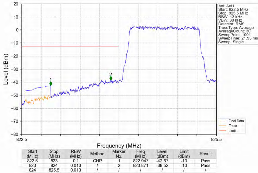
Band5 1.4MHz 64QAM LCH 824.7MHz RB 6 0 NTV
