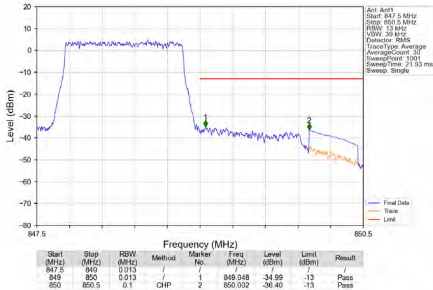
Band5 1.4MHz QPSK HCH 848.3MHz RB 6 0 NTV
