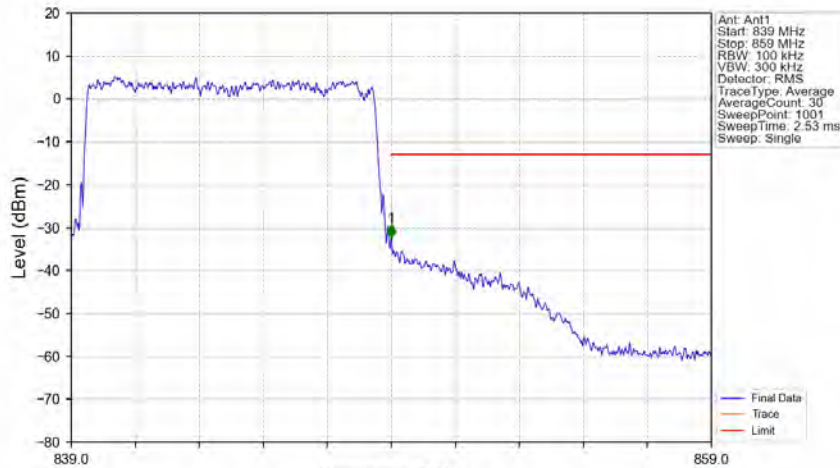
Band5_10MHz_QPSK_HCH_844MHz_RB_50_0_NTNV
