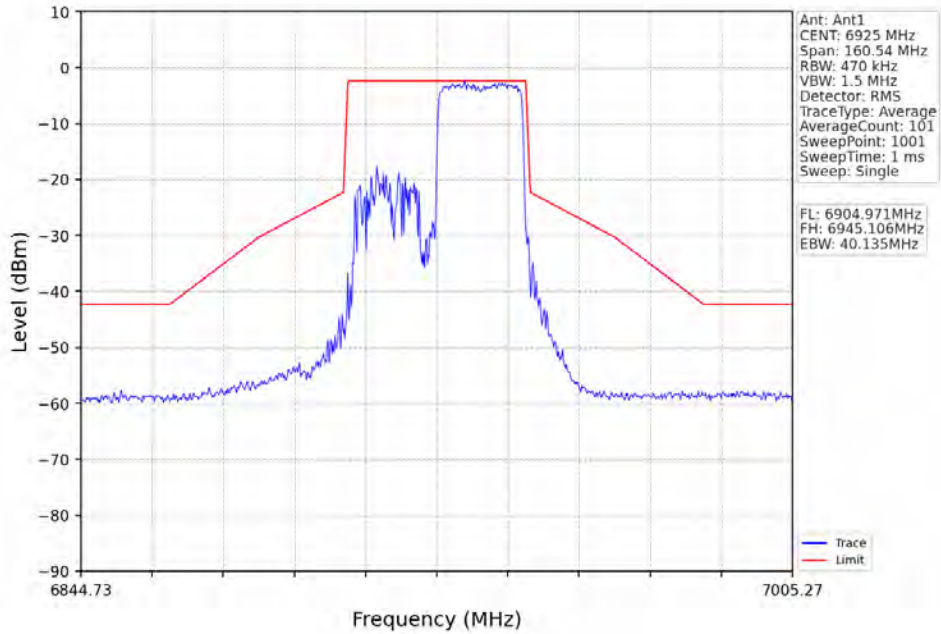
802.11ax(HE40)_LCH_6925MHz_RU484_Left_Ant1_NTNV
