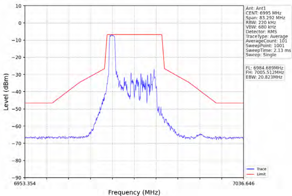
802.11ax(HE20)_MCH_6995MHz_RU26_Left_Ant1_NTNV
