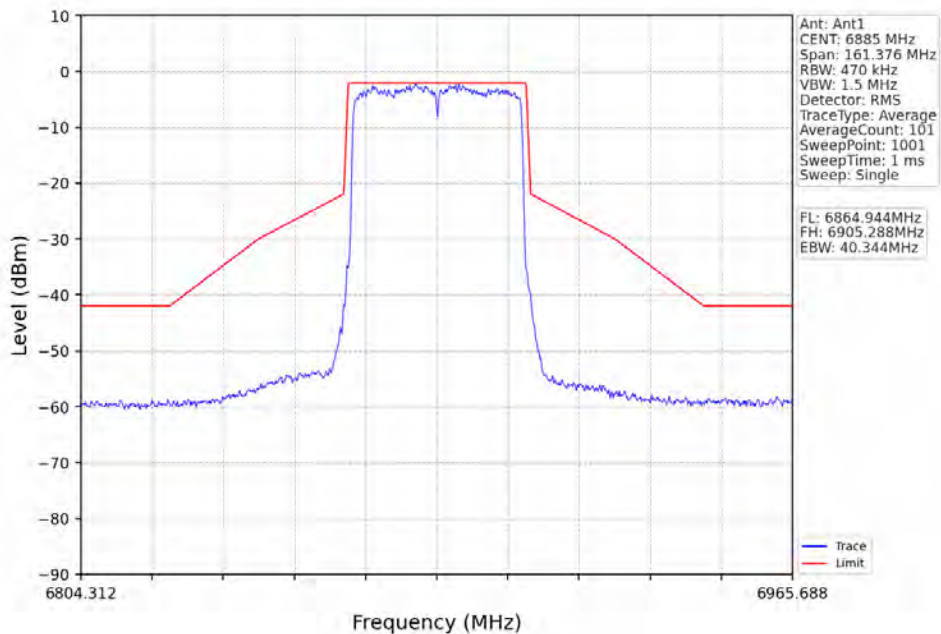
802.11ax(HE40)_HCH_6885MHz_RU484_Left_Ant1_NTNV
