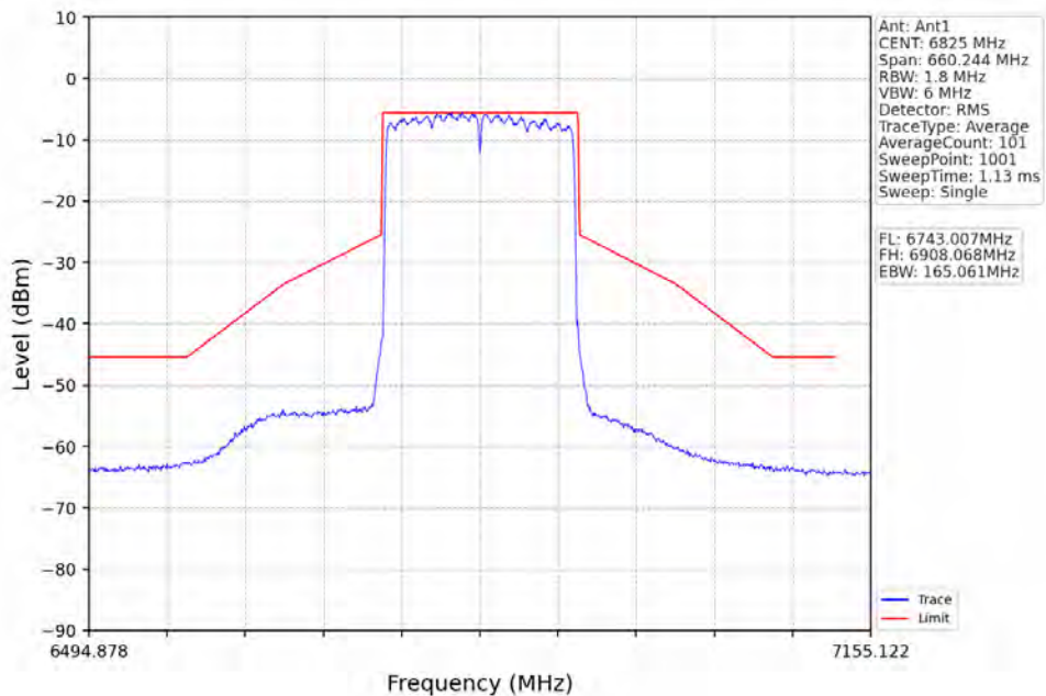
802.11ax(HE160)_HCH_6825MHz_2xRU996_Left_Ant1_NTNV
