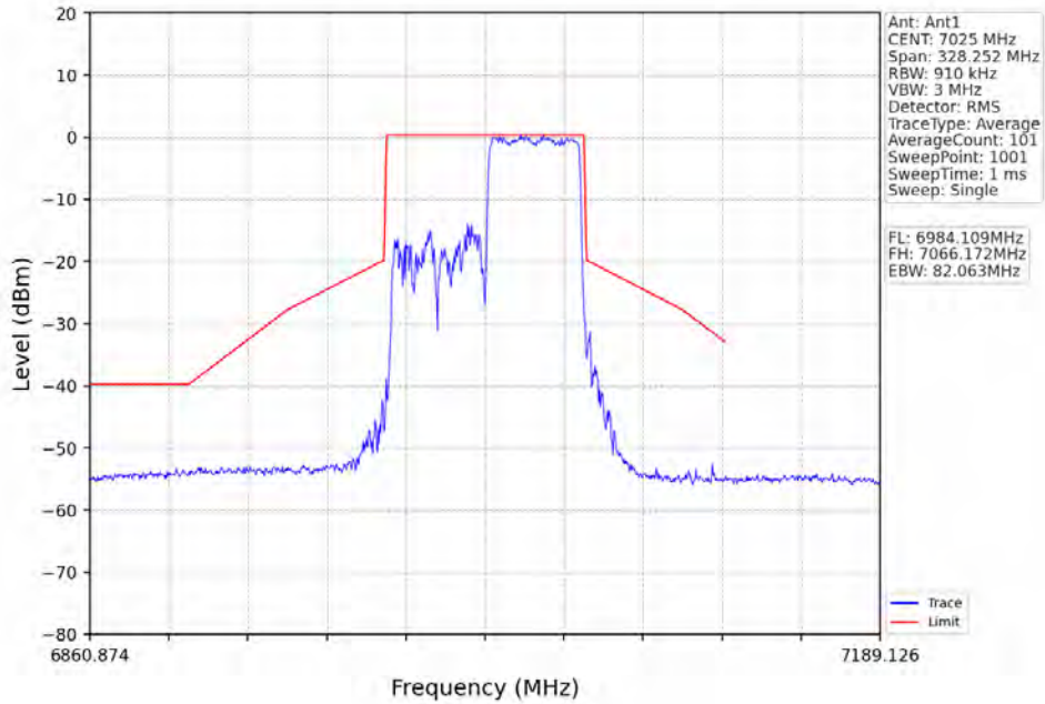
802.11ax(HE80)_HCH_7025MHz_RU996_Left_Ant1_NTNV
