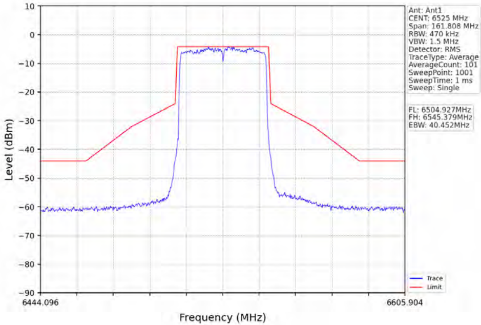
802.11ax(HE80)_HCH_6545MHz_RU484_Left_Ant1_NTNV
