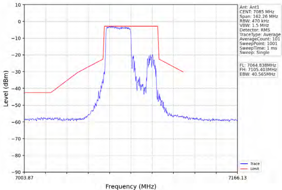
802.11ax(HE40)_HCH_7085MHz_RU242_Left_Ant1_NTNV
