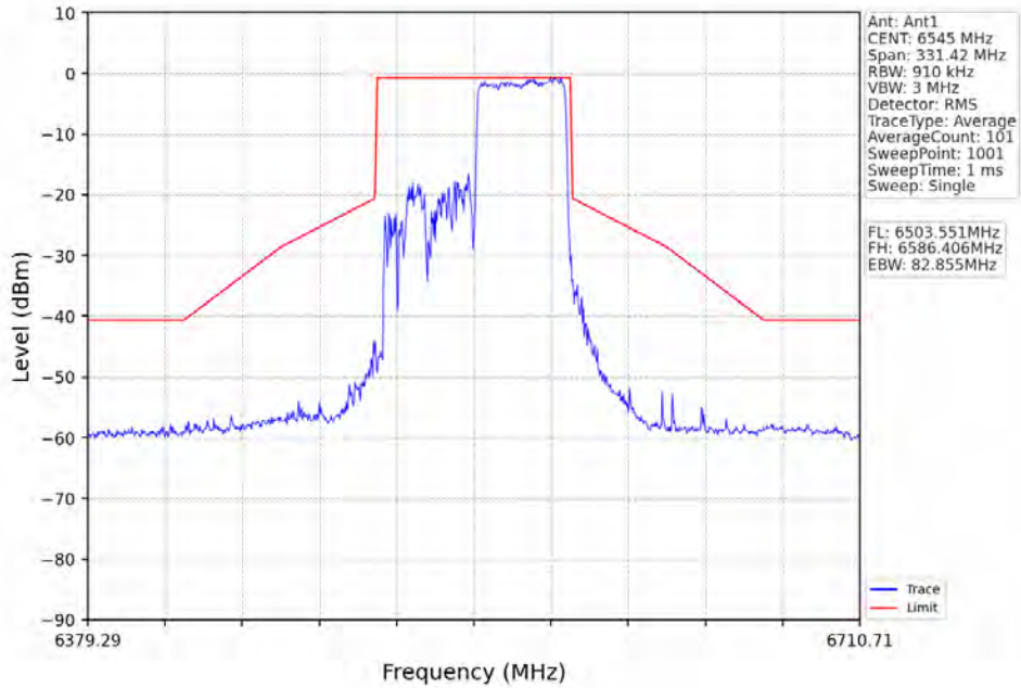
802.11ax(HE80)_HCH_6545MHz_RU996_Left_Ant1_NTNV
