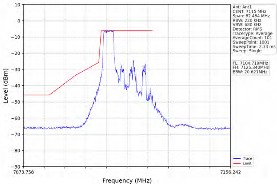
802.11ax(HE20)_HCH_7115MHz_RU52_Left_Ant1_NTNV
