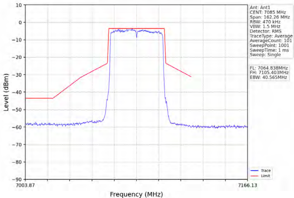
802.11ax(HE40)_HCH_7085MHz_RU484_Left_Ant1_NTNV
