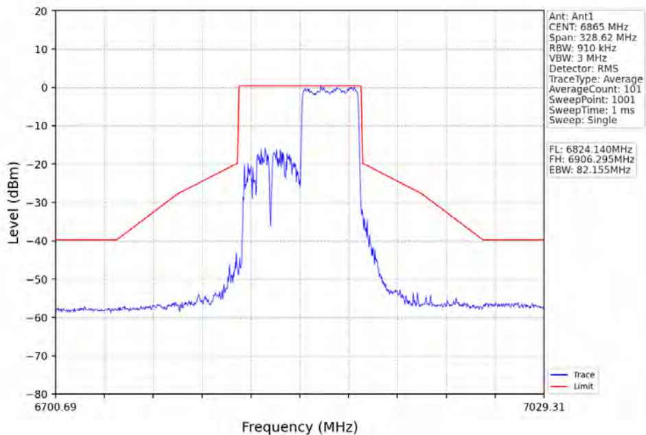
802.11ax(HE80)_HCH_6865MHz_RU484_Right_Ant1_NTNV
