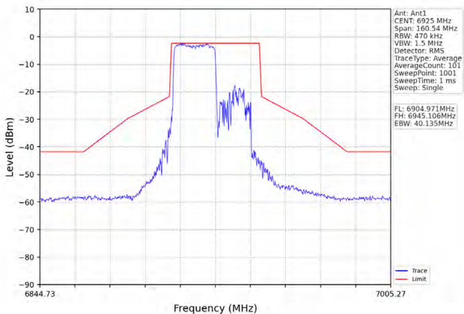
802.11ax(HE40)_LCH_6925MHz_RU242_Left_Ant1_NTNV
