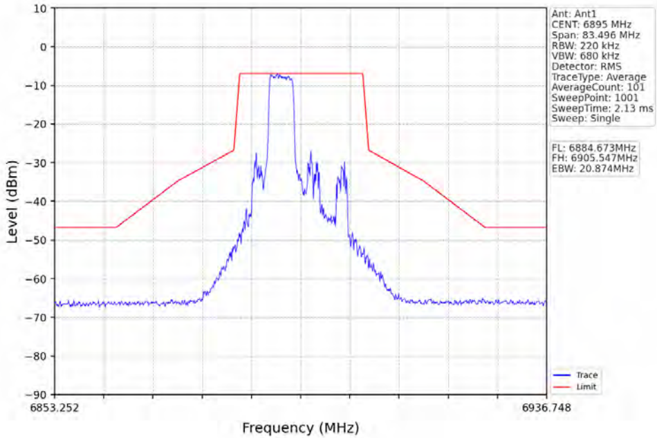
802.11ax(HE20)_LCH_6895MHz_RU52_Right_Ant1_NTNV
