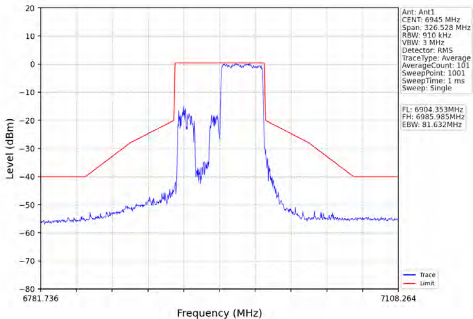
802.11ax(HE80)_LCH_6945MHz_RU484_Right_Ant1_NTNV
