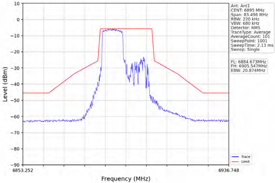
802.11ax(HE20)_LCH_6895MHz_RU106_Right_Ant1_NTNV
