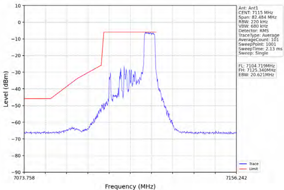
802.11ax(HE20)_HCH_7115MHz_RU52_Right_Ant1_NTNV
