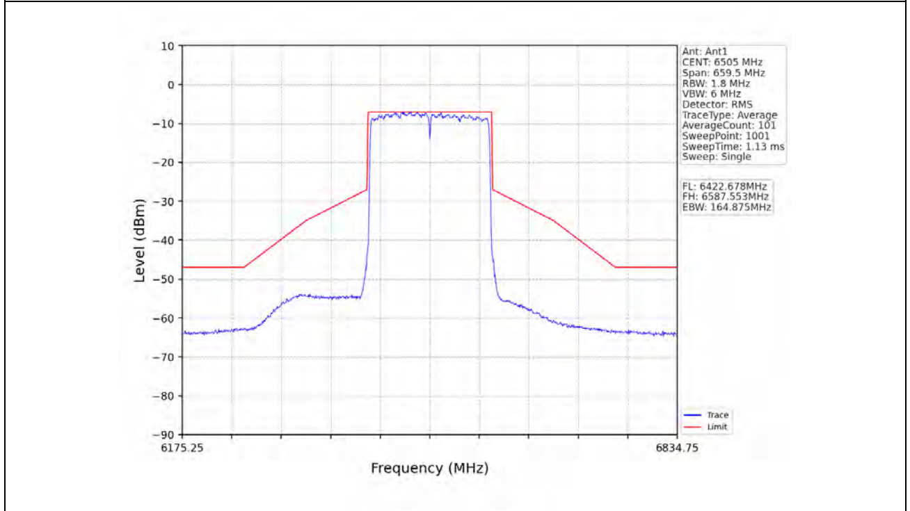
802.11ax(HE160)_HCH_6505MHz_2xRU996_Left_Ant1_NTNV
