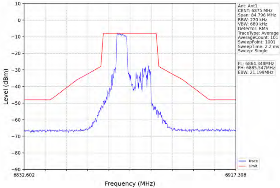
802.11ax(HE20)_HCH_6875MHz_RU52_Right_Ant1_NTNV
