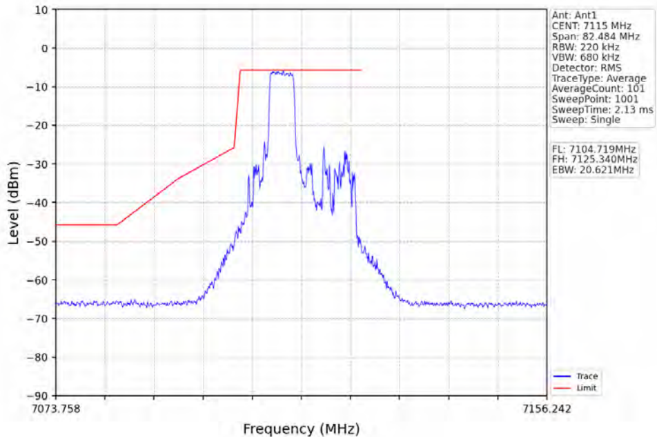
802.11ax(HE20)_HCH_7115MHz_RU52_Right_Ant1_NTNV
