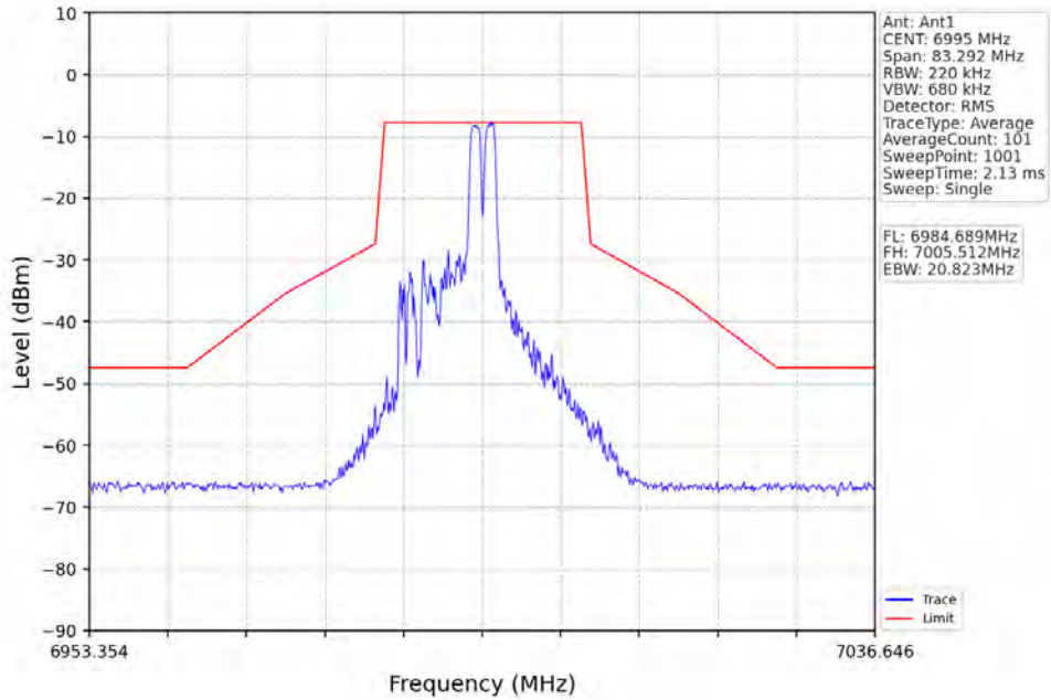
802.11ax(HE20)_MCH_6995MHz_RU26_Right_Ant1_NTNV
