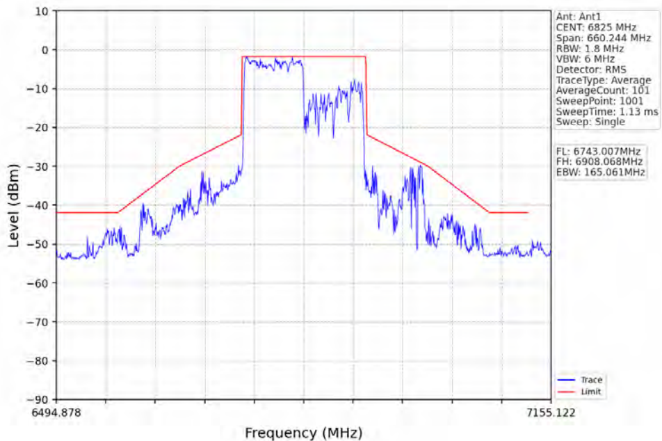
802.11ax(HE160)_HCH_6825MHz_RU996_Left_Ant1_NTNV
