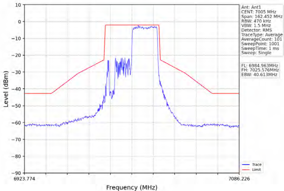
802.11ax(HE40)_MCH_7005MHz_RU242_Right_Ant1_NTNV
