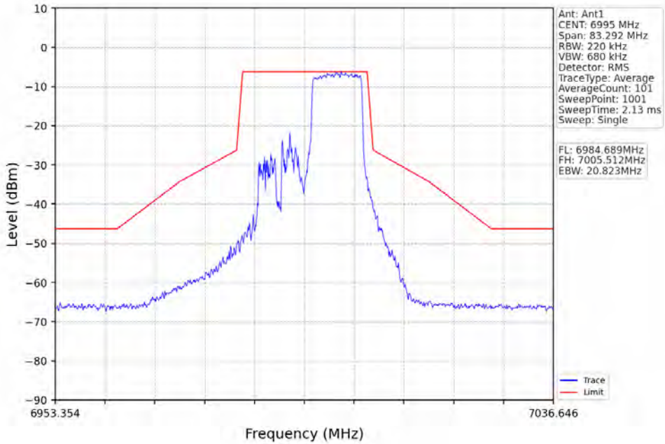
802.11ax(HE20)_MCH_6995MHz_RU242_Left_Ant1_NTNV
