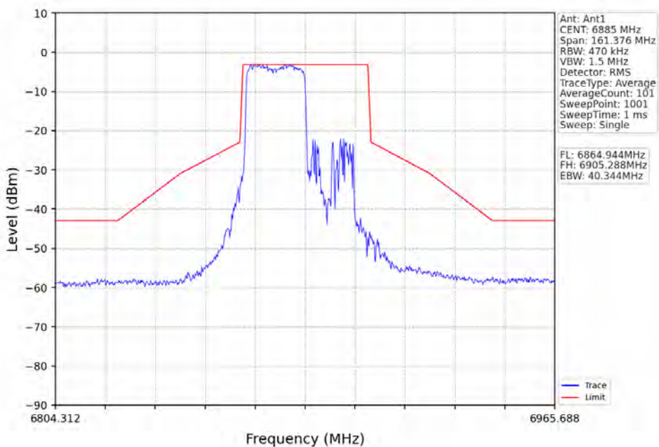
802.11ax(HE40)_HCH_6885MHz_RU242_Left_Ant1_NTNV
