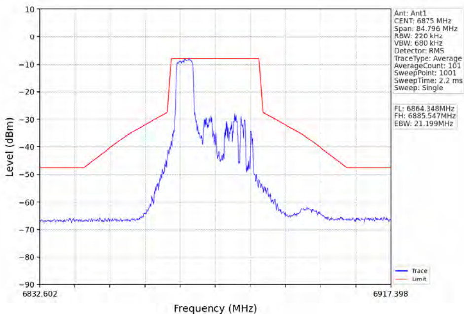
802.11ax(HE20)_HCH_6875MHz_RU52_Left_Ant1_NTNV
