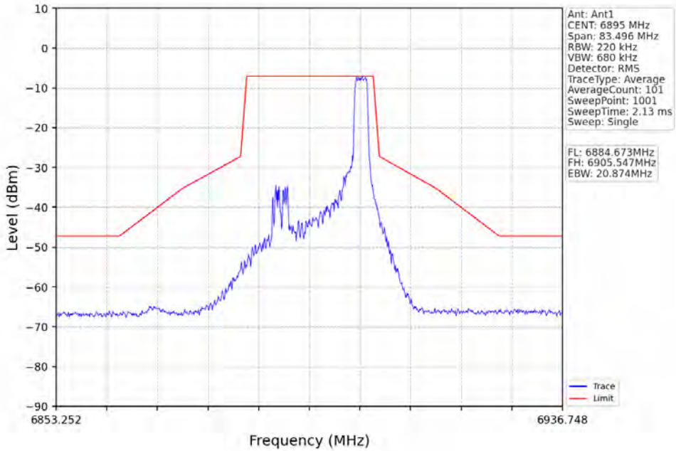
802.11ax(HE20)_LCH_6895MHz_RU52_Left_Ant1_NTNV
