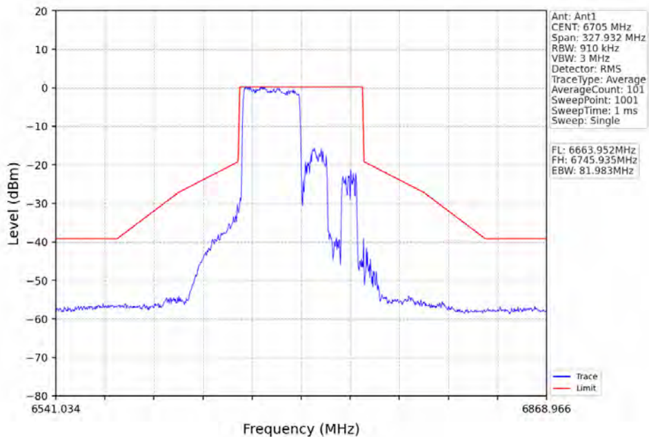
802.11ax(HE80)_MCH_6705MHz_RU484_Left_Ant1_NTNV
