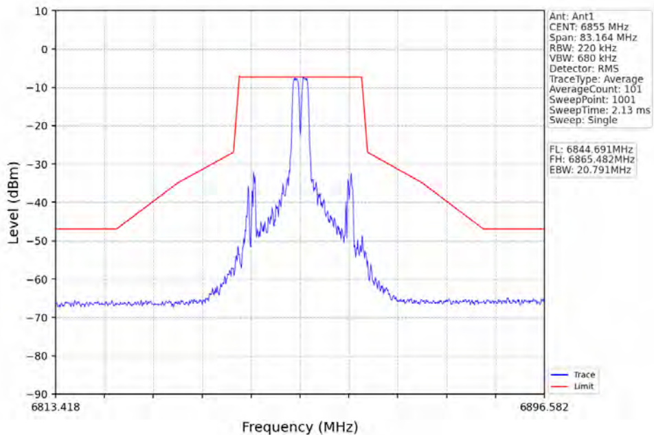
802.11ax(HE20)_HCH_6855MHz_RU26_Mid_Ant1_NTNV
