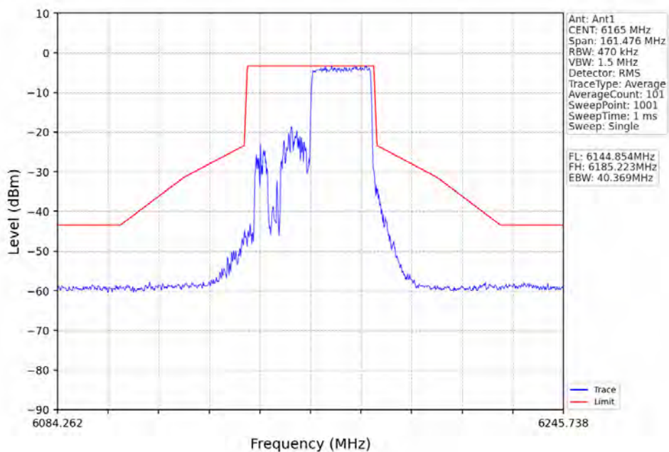
802.11ax(HE40)_MCH_6165MHz_RU242_Right_Ant1_NTNV
