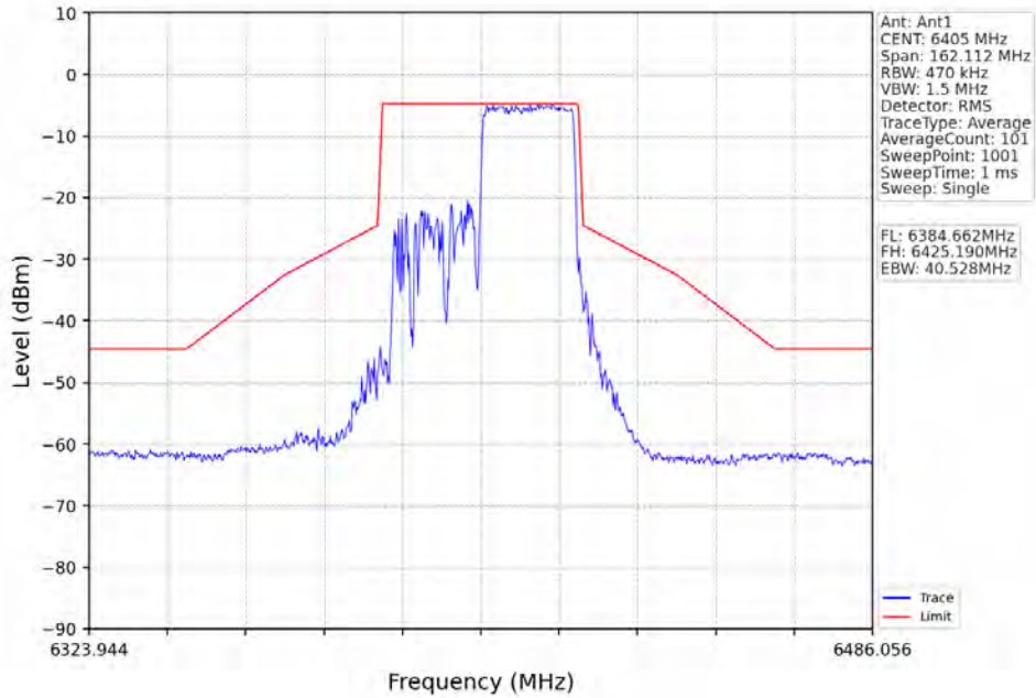
802.11ax(HE40)_HCH_6405MHz_RU484_Left_Ant1_NTNV
