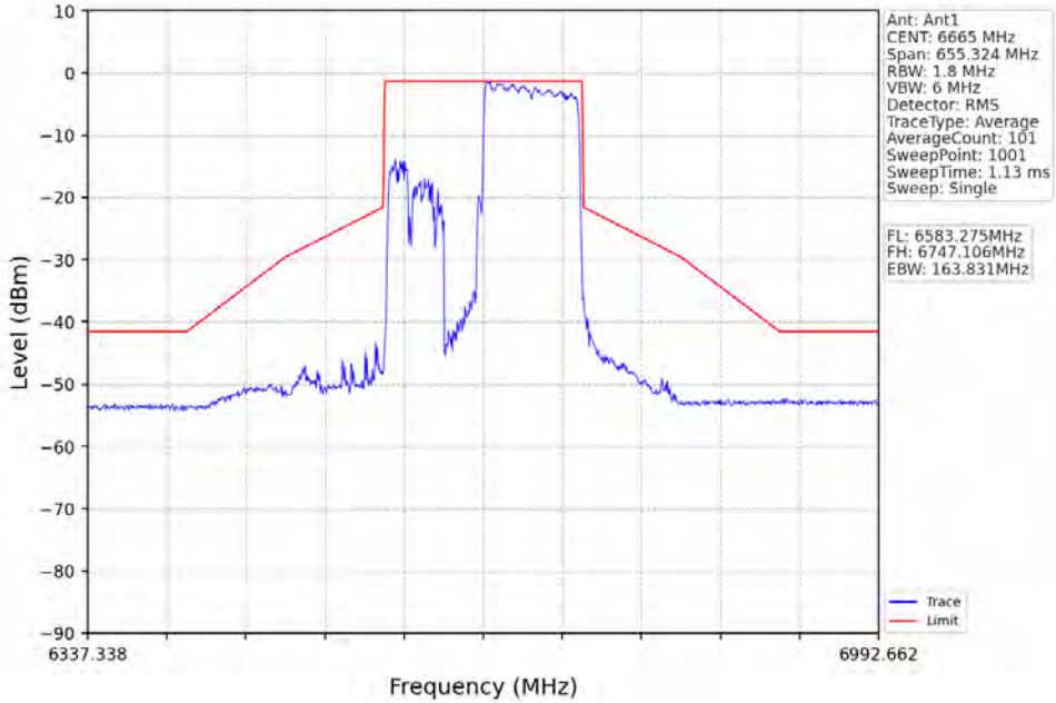
802.11ax(HE160)_MCH_6665MHz_2xRU996_Left_Ant1_NTNV
