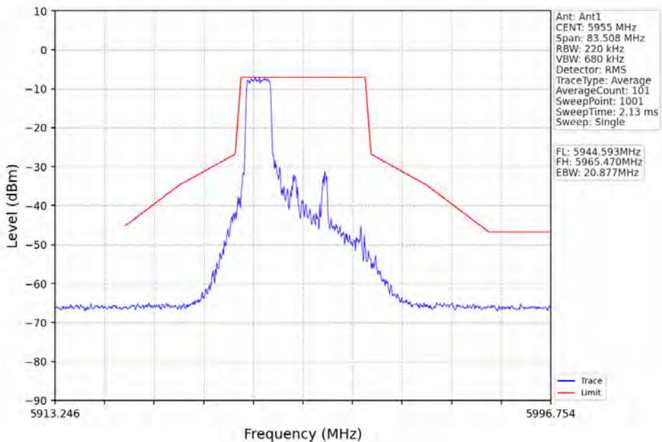
802.11ax(HE20)_LCH_5955MHz_RU52_Left_Ant1_NTNV
