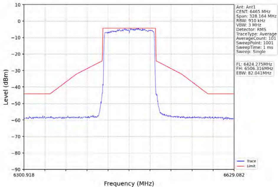
802.11ax(HE80)_LCH_6465MHz_RU996_Left_Ant1_NTNV
