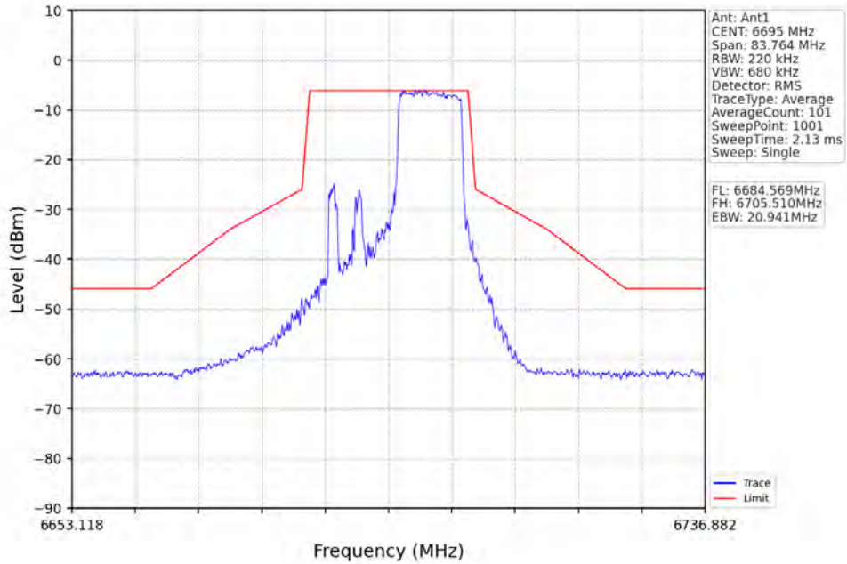
802.11ax(HE20)_MCH_6695MHz_RU242_Left_Ant1_NTNV
