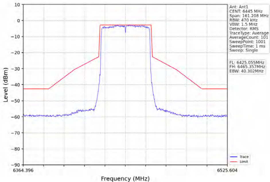
802.11ax(HE40)_LCH_6445MHz_RU484_Left_Ant1_NTNV
