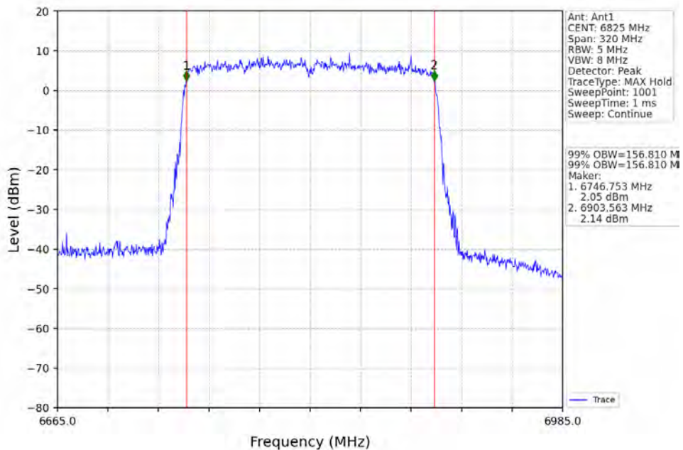
802.11ax(HE160)_HCH_6825MHz_2xRU996_Left_Ant1_NTNV
