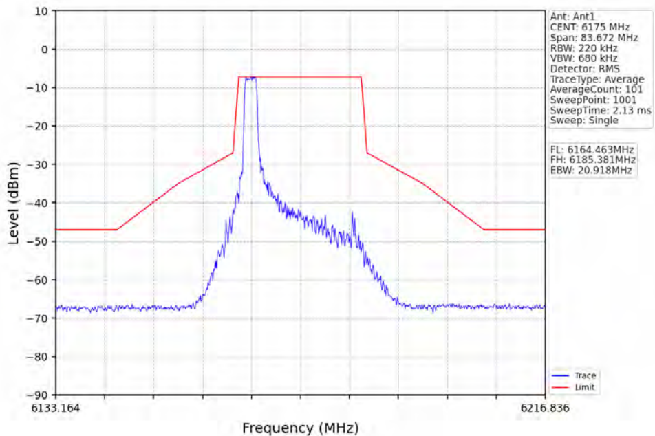
802.11ax(HE20)_MCH_6175MHz_RU26_Left_Ant1_NTNV
