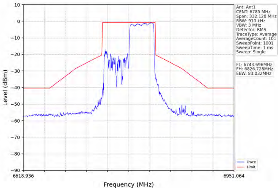
802.11ax(HE80)_HCH_6785MHz_RU484_Right_Ant1_NTNV
