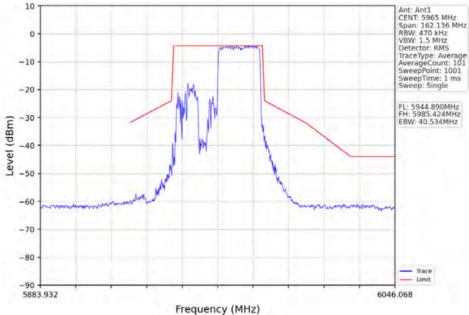
802.11ax(HE40)_LCH_5965MHz_RU484_Left_Ant1_NTNV
