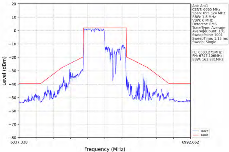
802.11ax(HE160)_MCH_6665MHz_RU996_Left_Ant1_NTNV
