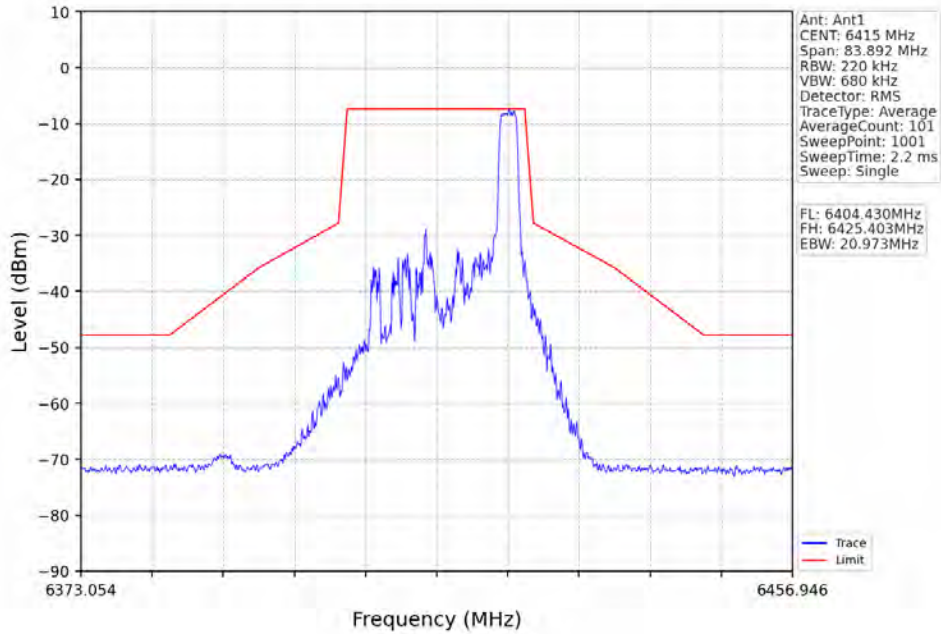
802.11ax(HE20)_HCH_6415MHz_RU52_Left_Ant1_NTNV
