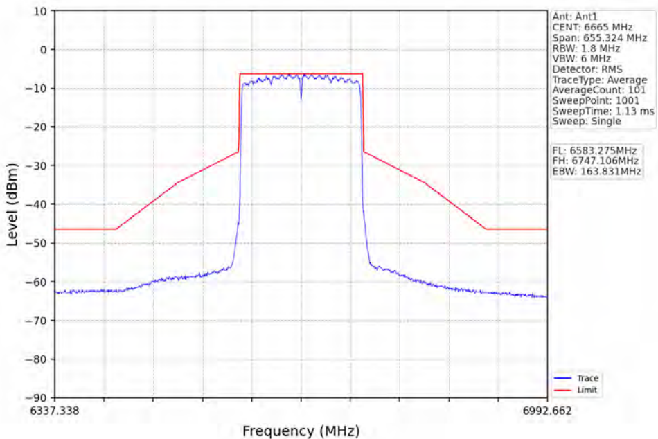
802.11ax(HE160)_MCH_6665MHz_2xRU996_Left_Ant1_NTNV
