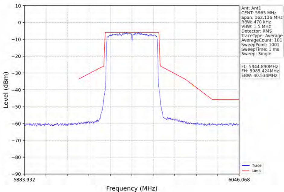
802.11ax(HE40)_LCH_5965MHz_RU484_Left_Ant1_NTNV
