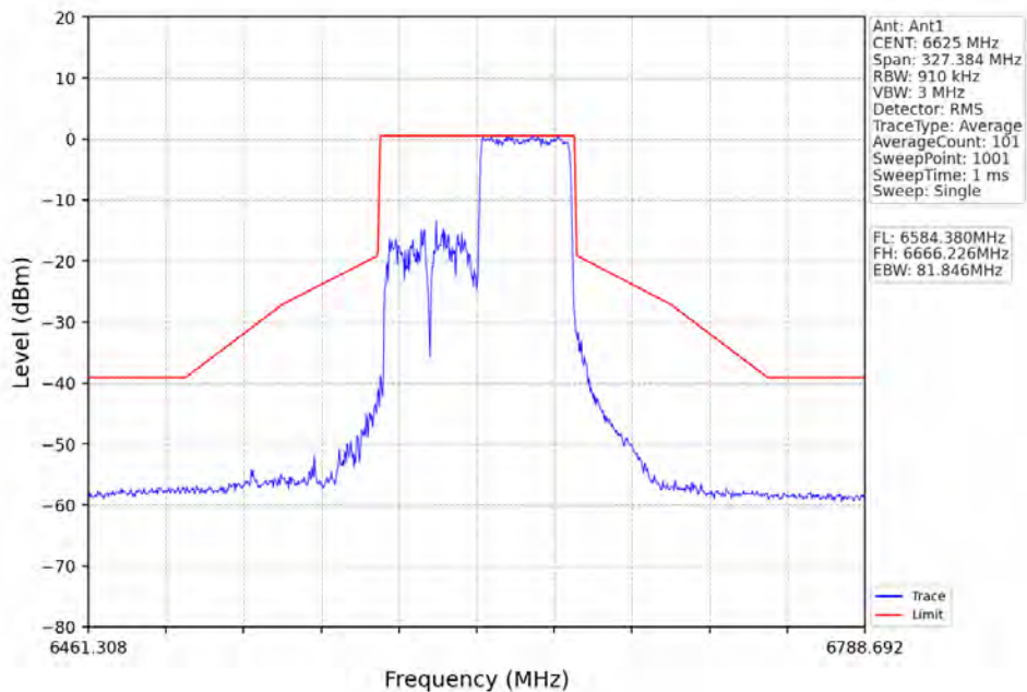
802.11ax(HE80)_LCH_6625MHz_RU484_Right_Ant1_NTNV
