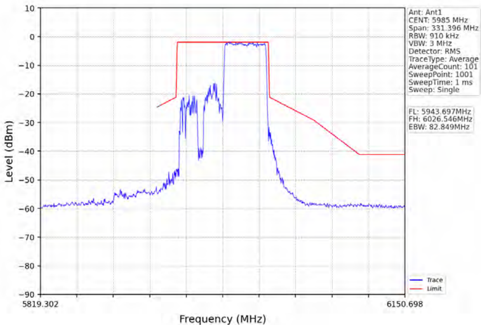
802.11ax(HE80)_LCH_5985MHz_RU484_Right_Ant1_NTNV
