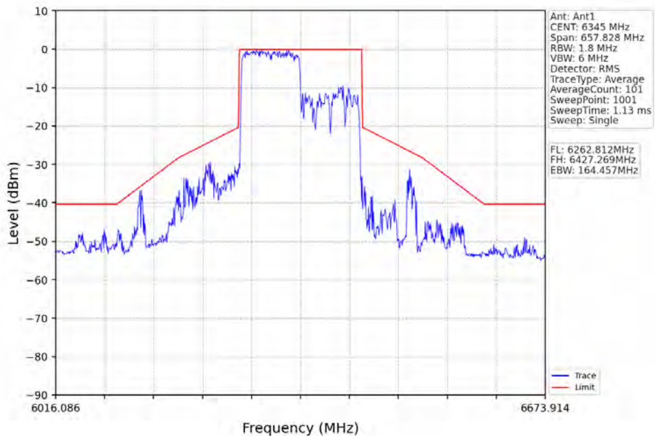
802.11ax(HE160)_HCH_6345MHz_RU996_Left_Ant1_NTNV
