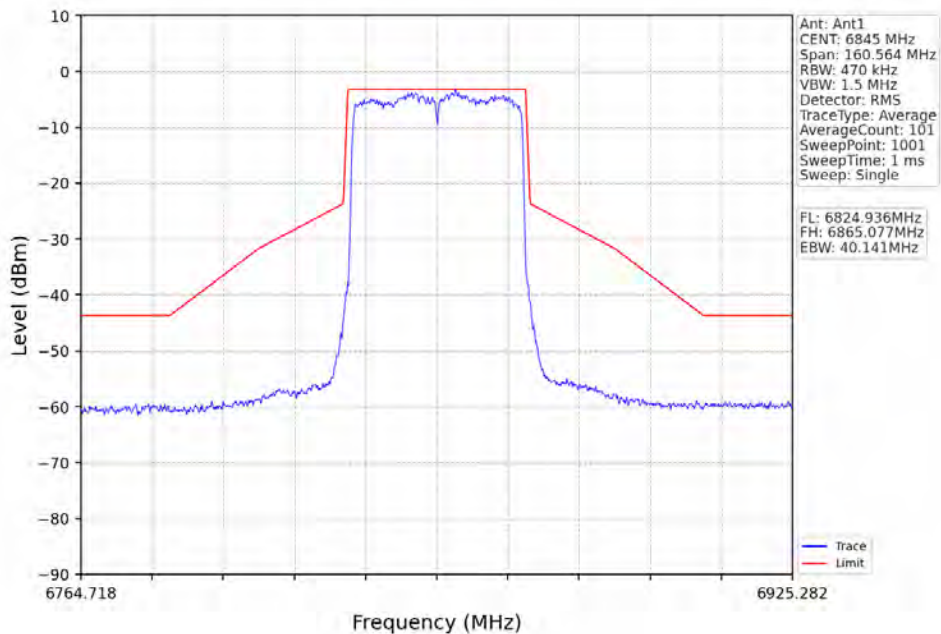
802.11ax(HE40)_HCH_6845MHz_RU484_Left_Ant1_NTNV
