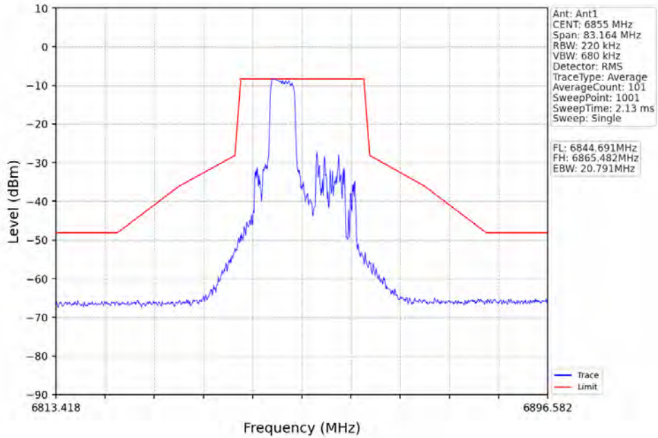
802.11ax(HE20)_HCH_6855MHz_RU52_Right_Ant1_NTNV
