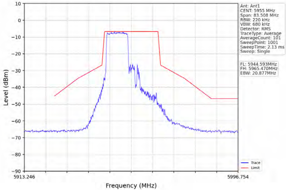
802.11ax(HE20)_LCH_5955MHz_RU106_Right_Ant1_NTNV
