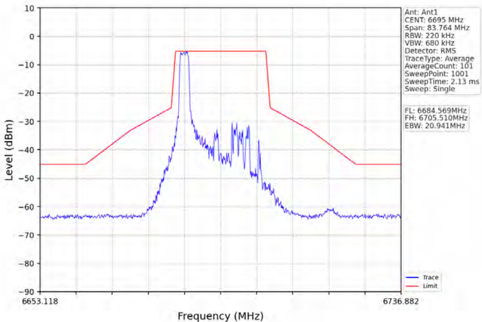
802.11ax(HE20)_MCH_6695MHz_RU26_Left_Ant1_NTNV
