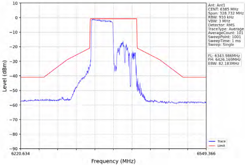
802.11ax(HE80)_HCH_6385MHz_RU484_Right_Ant1_NTNV
