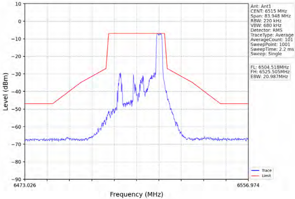
802.11ax(HE20)_HCH_6515MHz_RU52_Left_Ant1_NTNV
