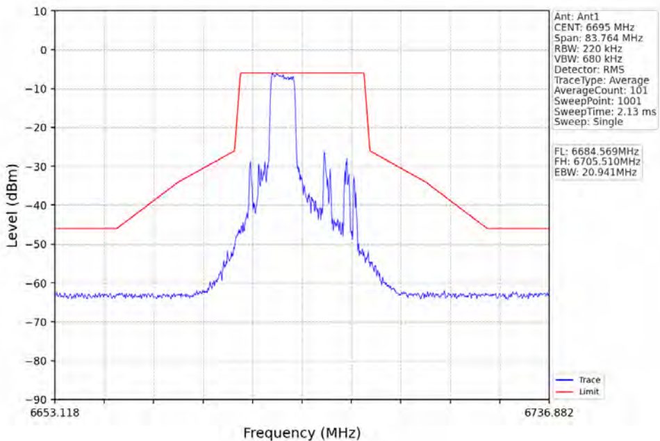
802.11ax(HE20)_MCH_6695MHz_RU52_Mid_Ant1_NTNV
