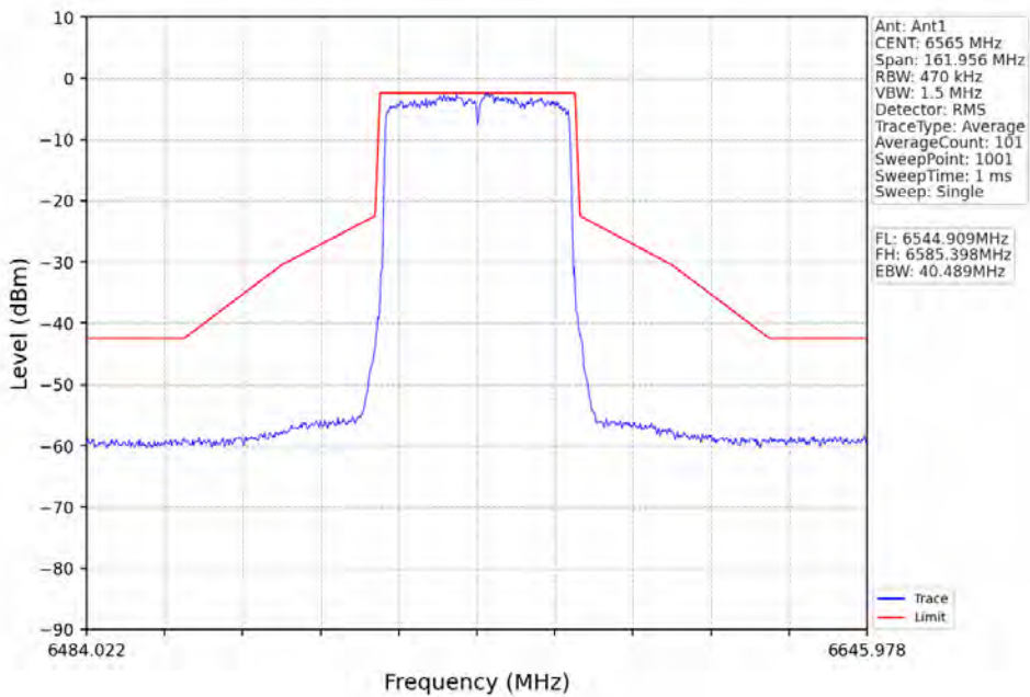
802.11ax(HE40)_LCH_6565MHz_RU484_Left_Ant1_NTNV
