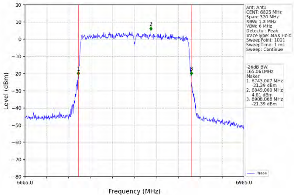
802.11ax(HE160)_HCH_6825MHz_2xRU996_Left_Ant1_NTNV
