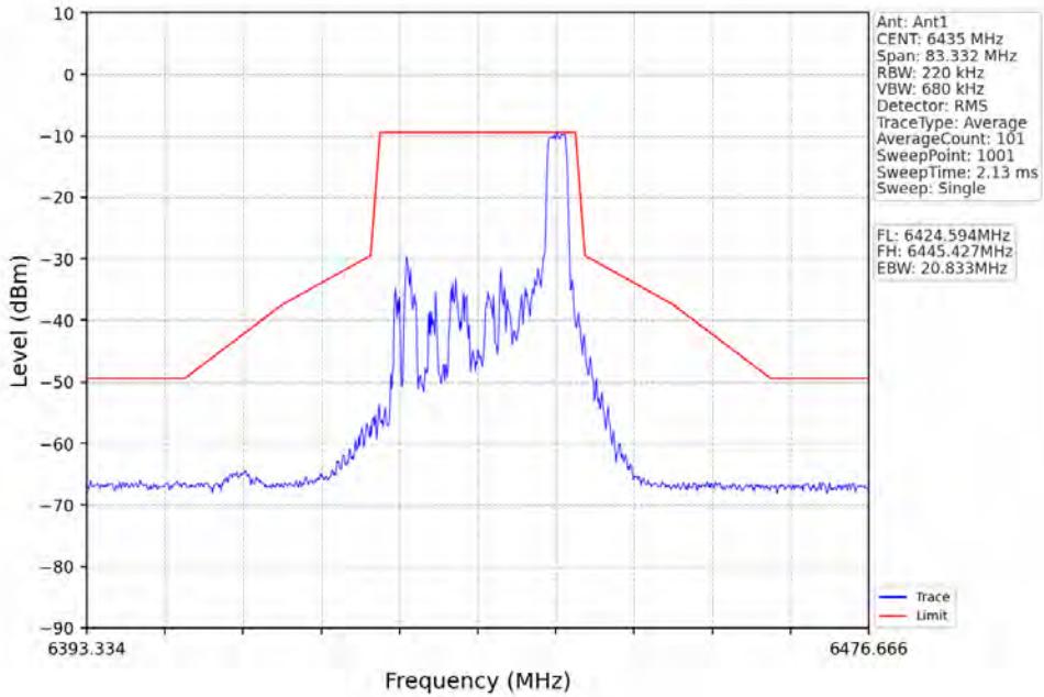
802.11ax(HE20)_LCH_6435MHz_RU52_Left_Ant1_NTNV
