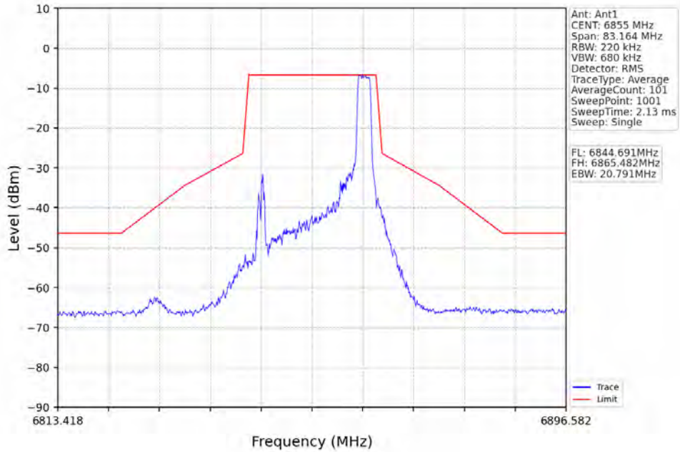
802.11ax(HE20)_HCH_6855MHz_RU52_Left_Ant1_NTNV
