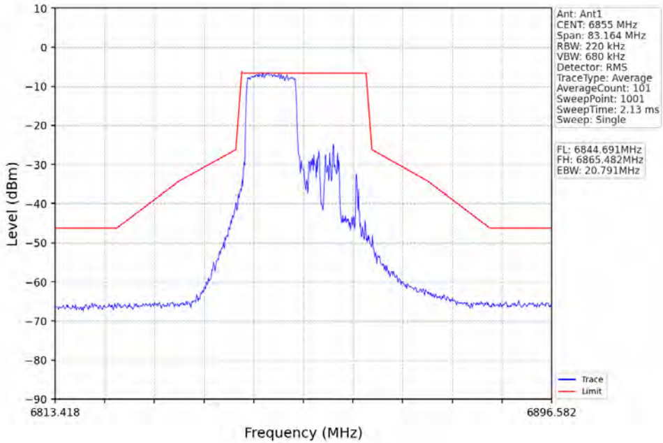
802.11ax(HE20)_HCH_6855MHz_RU106_Right_Ant1_NTNV
