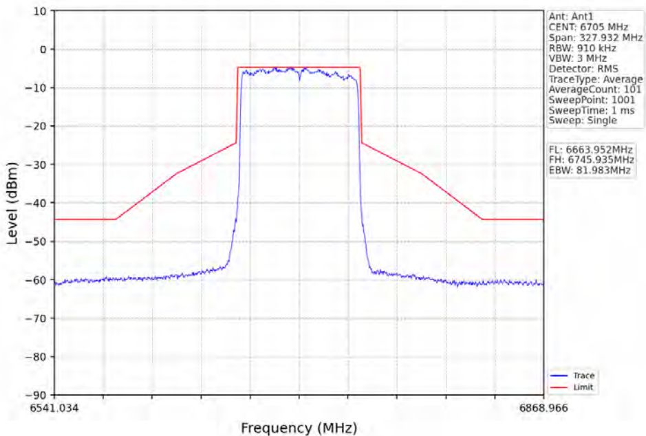
802.11ax(HE80)_MCH_6705MHz_RU996_Left_Ant1_NTNV
