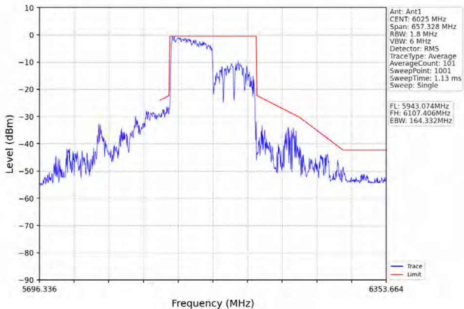
802.11ax(HE160)_LCH_6025MHz_RU996_Left_Ant1_NTNV
