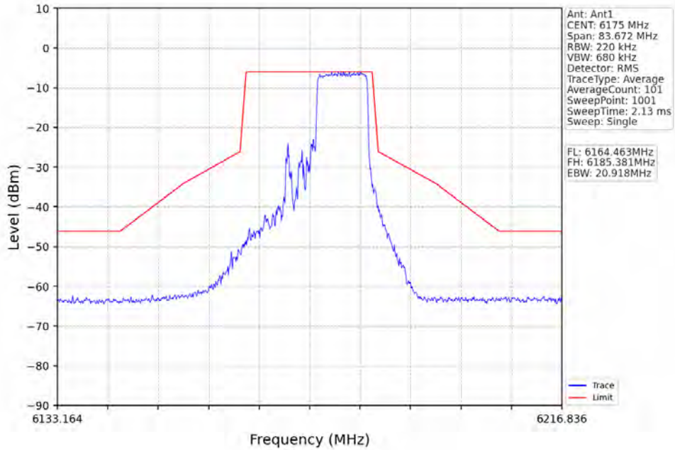
802.11ax(HE20)_MCH_6175MHz_RU242_Left_Ant1_NTNV
