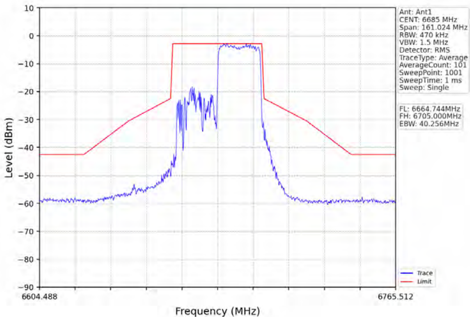
802.11ax(HE40)_MCH_6685MHz_RU242_Right_Ant1_NTNV
