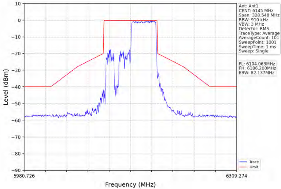
802.11ax(HE80)_MCH_6145MHz_RU996_Left_Ant1_NTNV
