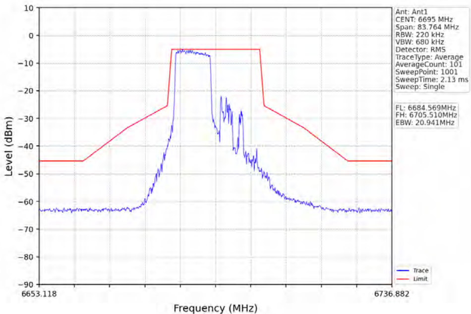
802.11ax(HE20)_MCH_6695MHz_RU106_Left_Ant1_NTNV
