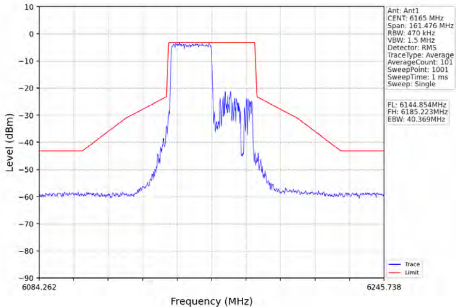
802.11ax(HE40)_MCH_6165MHz_RU242_Right_Ant1_NTNV
