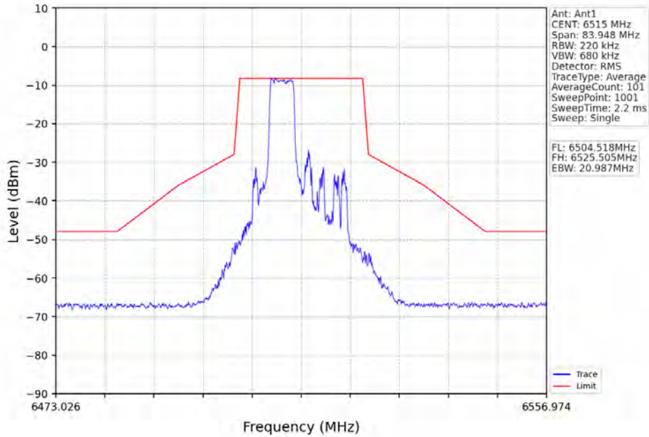
802.11ax(HE20)_HCH_6515MHz_RU52_Right_Ant1_NTNV
