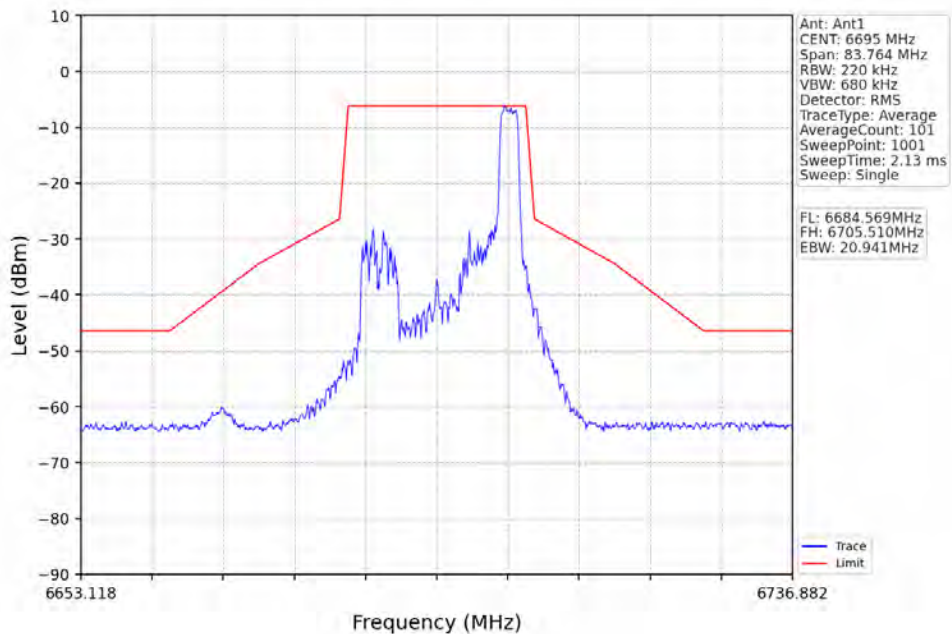
802.11ax(HE20)_MCH_6695MHz_RU26_Right_Ant1_NTNV
