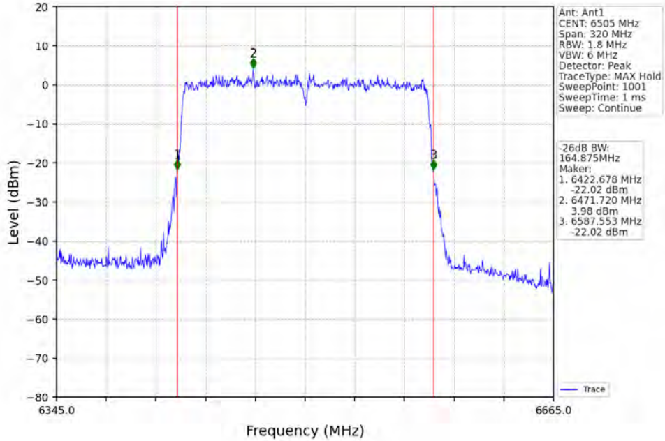
802.11ax(HE160)_HCH_6505MHz_2xRU996_Left_Ant1_NTNV
