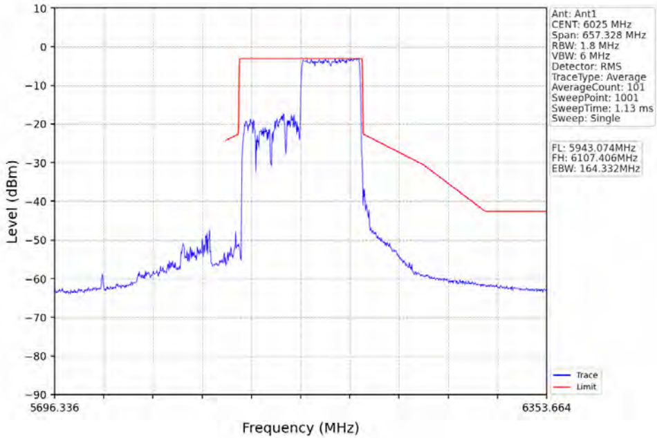
802.11ax(HE160)_LCH_6025MHz_2xRU996_Left_Ant1_NTNV
