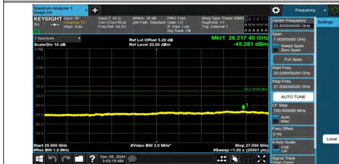
Band41-20MHz-QPSK-39750-1RB#0-20000~27000-PASS
