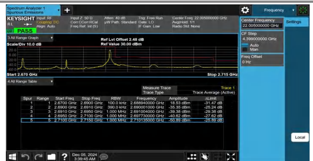
Band41-20MHz-QPSK-41490-1RB#99-PASS
