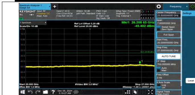
Band41-15MHz-QPSK-39725-1RB#0-20000~27000-PASS
