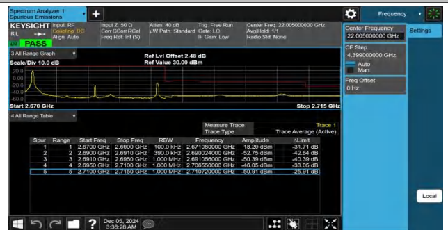
Band41-20MHz-QPSK-41490-1RB#0-PASS
