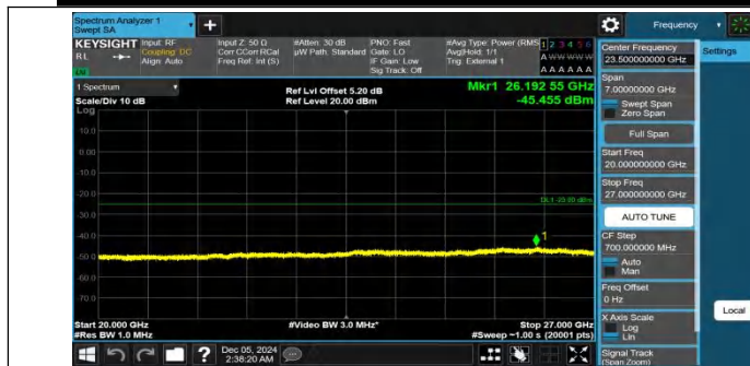
Band41-5MHz-QPSK-41565-1RB#0-20000~27000-PASS
