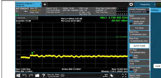
Band26(824-849)-10MHz-QPSK-26990-1RB#0-3000~10000-PAS
