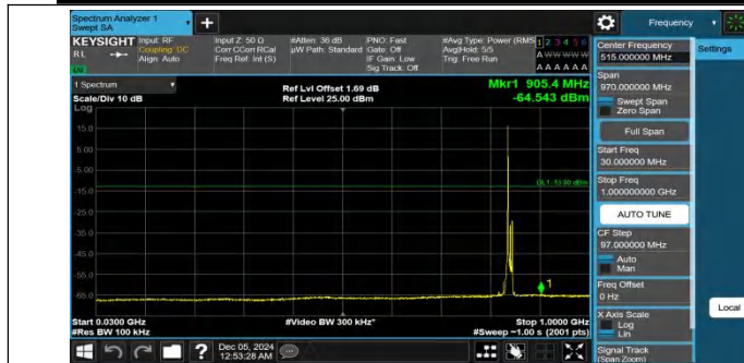
Band26(824-849)-10MHz-QPSK-26990-1RB#0-30~1000-PASS
