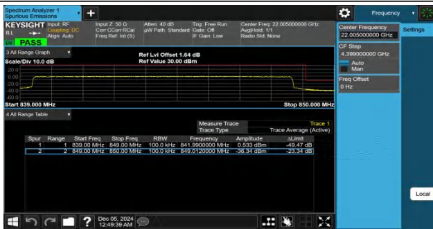
Band26(824-849)-10MHz-QPSK-26990-50RB#0-PASS
