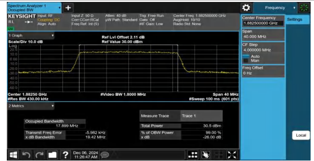
Band25-20MHz-16QAM-26365-100RB#0-PASS
