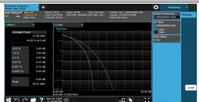
Band25-10MHz-16QAM-26365-50RB#0-PASS
