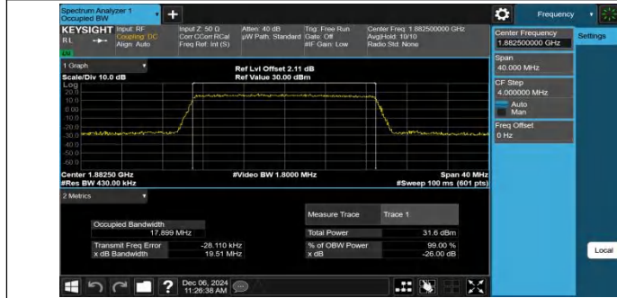
Band25-20MHz-QPSK-26365-100RB#0-PASS
