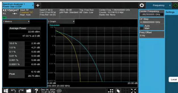
Band25-20MHz-QPSK-26365-100RB#0-PASS
