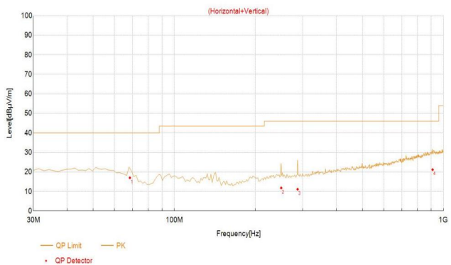
WIFI_2.4G_11b_20M_2462
