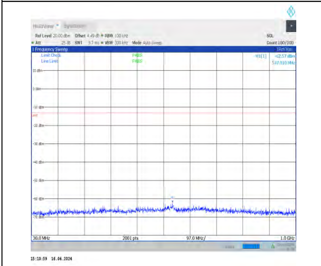
1-N78-3700-3800-N78-3700-380030-100-H-1-DFT-P I2BPSK-Inner_1RB_Left-1@1-30-1000-Ant1-677.96 --62.57--13-PASS
