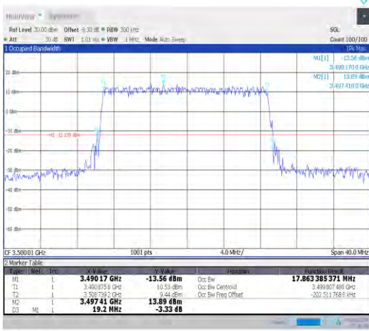
1-N78-3450-3550-30-20-M-5-DFT-256QAM-Outer_Full ull-50@0-Ant1-17.863-19.200-≤20-PASS
