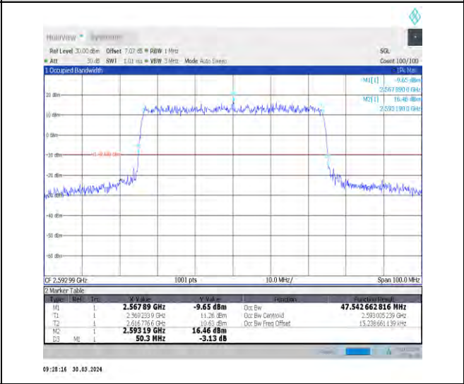
1-N41-30-50-M-6-CP-QPSK-Outer_Full-133@0-Ant1 -47.543-50.300-≤50-PASS
