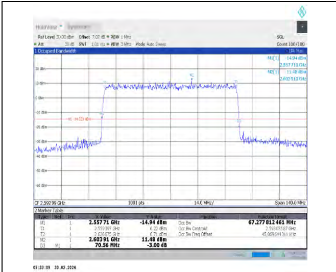
1-N41-30-70-M-9-CP-256QAM-Outer_Full-189@0-A nt1-67.278-70.560-≤70-PASS
