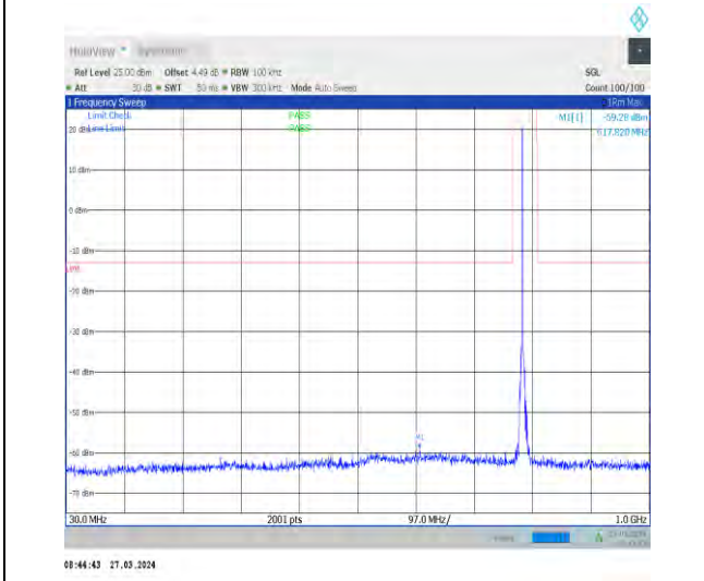
1-N14-15-10-H-1-DFT-PI2BPSK-Inner_1RB_Left-1 @1-30-1000-Ant1-617.82--59.28--13-PASS
