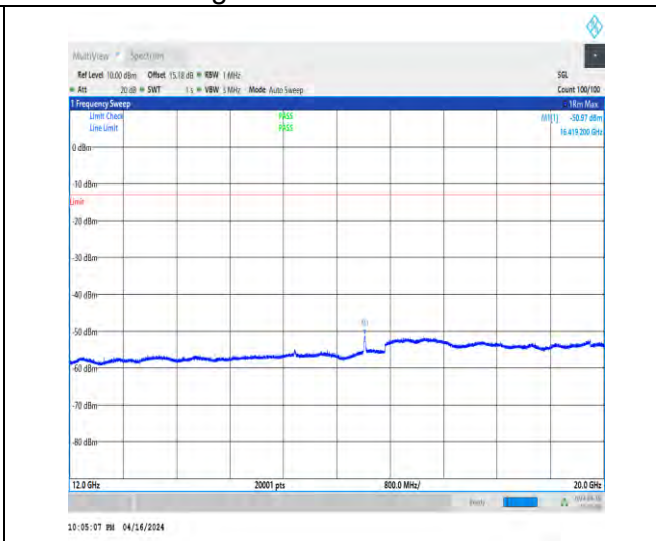
1-N5-15-20-L-1-DFT-QPSK-Edge_1RB_Left-1@0-12 000-20000-Ant1-16419.20--50.97--13-PASS
