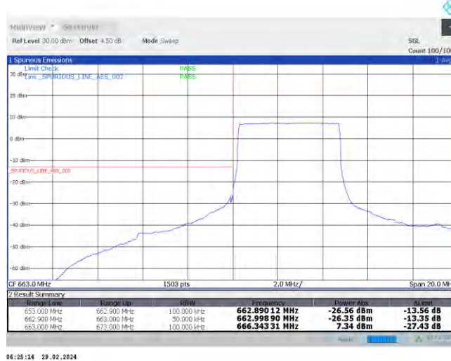
Band71-5MHz-QPSK-133147-25RB#0
