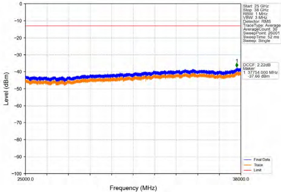
Band43d_20MHz_QPSK_LCH_3710MHz_RB_100_0_NTNV
