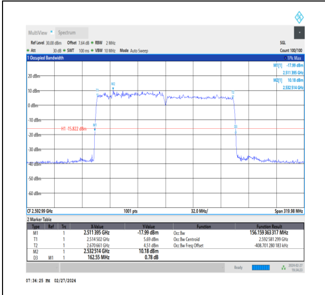
NTVN_CA_n41C_PC3_30+30_80+80_M+M_Ant1_TID3_1_#1
