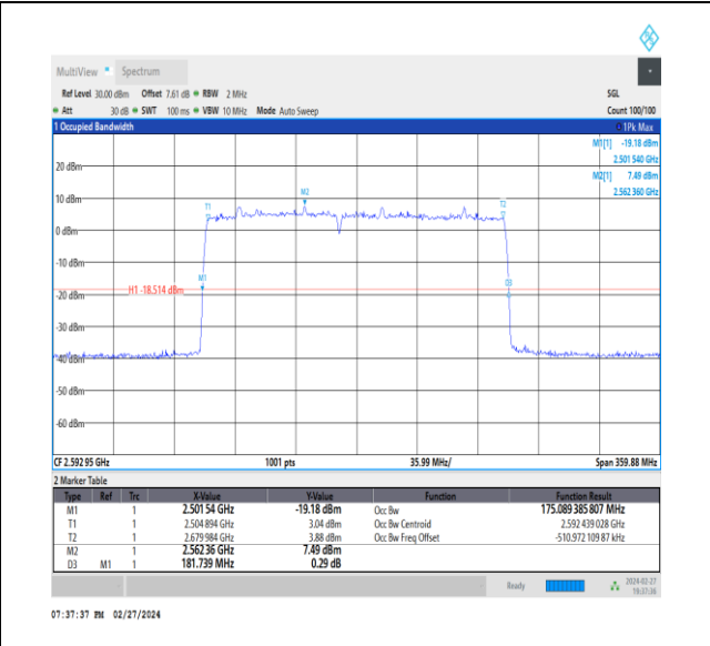
NTVN_CA_n41C_PC3_30+30_80+100_M+M_Ant1_TID1_1_#1
