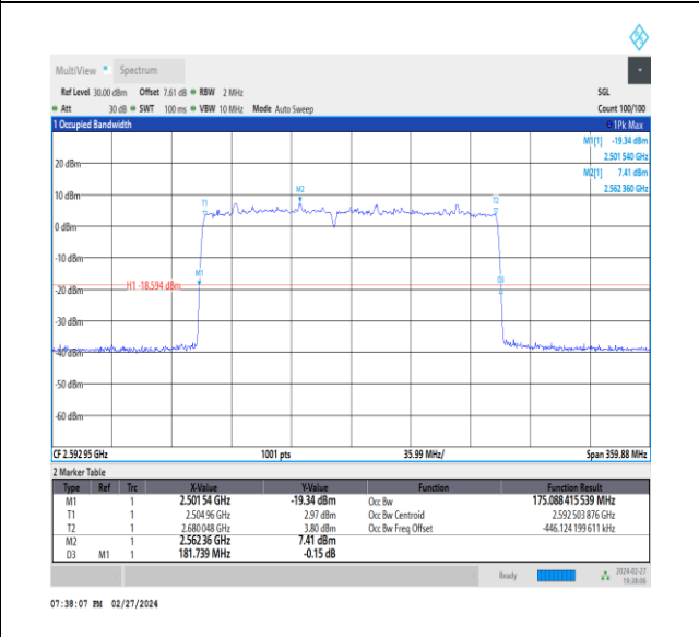
NTVN_CA_n41C_PC3_30+30_80+100_M+M_Ant1_TID3_1_#1
