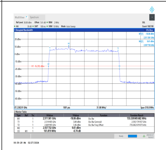
NTNV_CA_n41C_PC3_30+30_60+100_M+M_Ant1_TID1_1_#1
