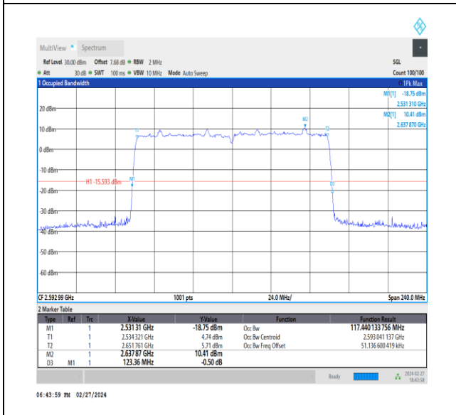
NTVN_CA_n41C_PC3_30+30_60+60_M+M_Ant1_TID2_1_#1
