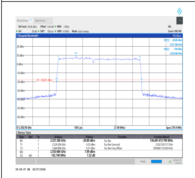
NTNV_CA_n41C_PC3_30+30_60+80_M+M_Ant1_TID5_1_#1
