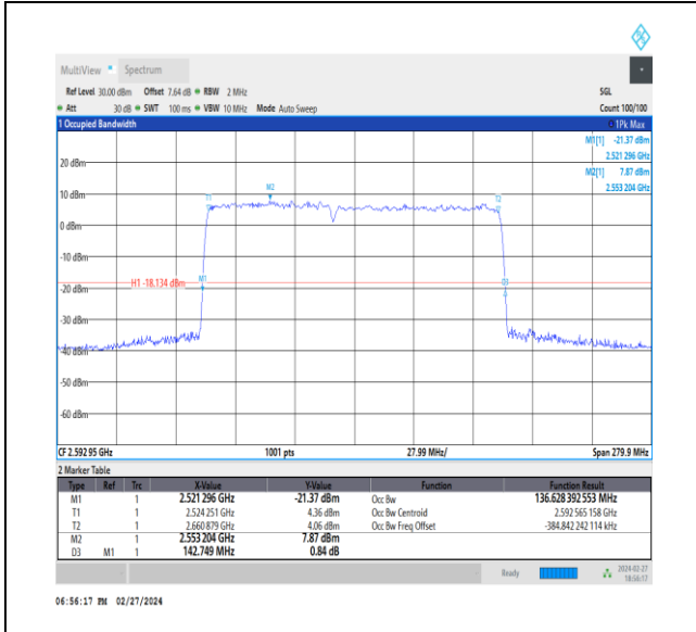
NTNV_CA_n41C_PC3_30+30_60+80_M+M_Ant1_TID3_1_#1
