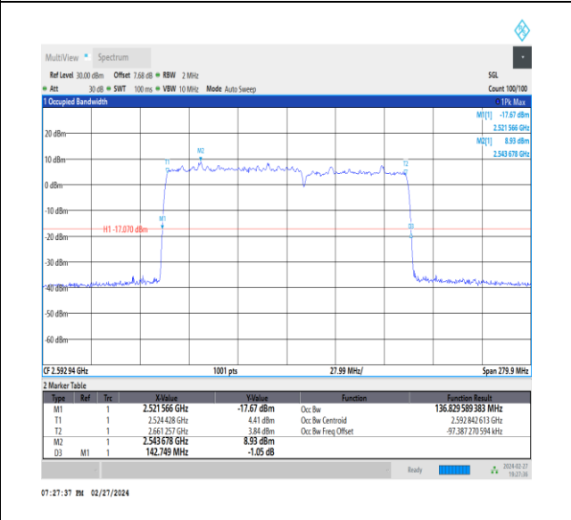
NTVN_CA_n41C_PC3_30+30_80+60_M+M_Ant1_TID4_1_#1
