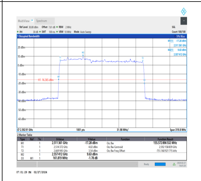
NTNV_CA_n41C_PC3_30+30_60+100_M+M_Ant1_TID9 _1_#1
