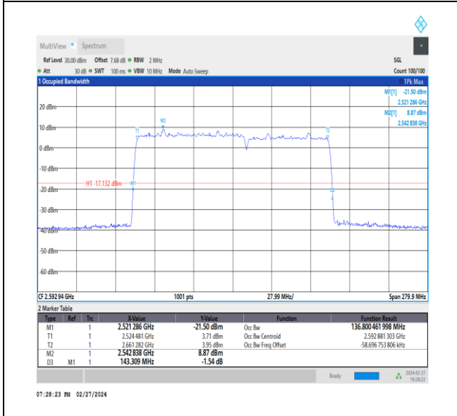
NTNV_CA_n41C_PC3_30+30_80+60_M+M_Ant1_TID7_1_#1
