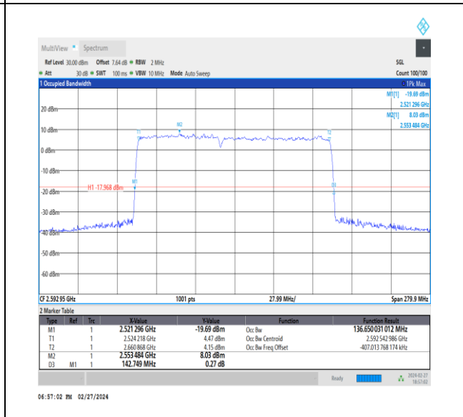
NTNV_CA_n41C_PC3_30+30_60+80_M+M_Ant1_TID6_1_#1
