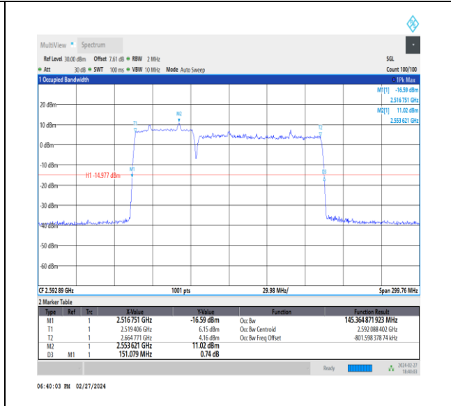
NTVN_CA_n41C_PC3_30+30_50+100_M+M_Ant1_TID2_1_#1
