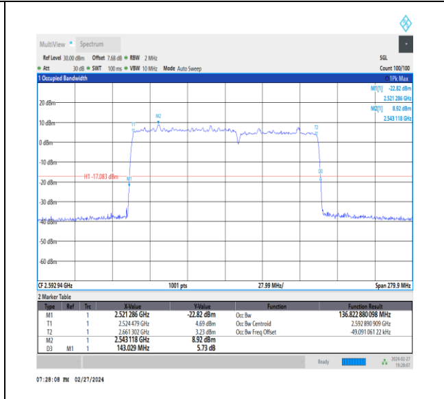
NTNV_CA_n41C_PC3_30+30_80+60_M+M_Ant1_TID6_1_#1
