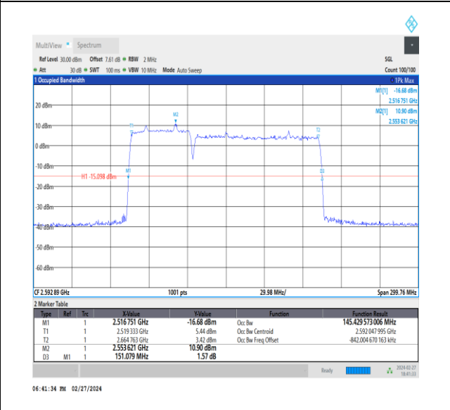
NTVN_CA_n41C_PC3_30+30_50+100_M+M_Ant1_TID8_1_#1
