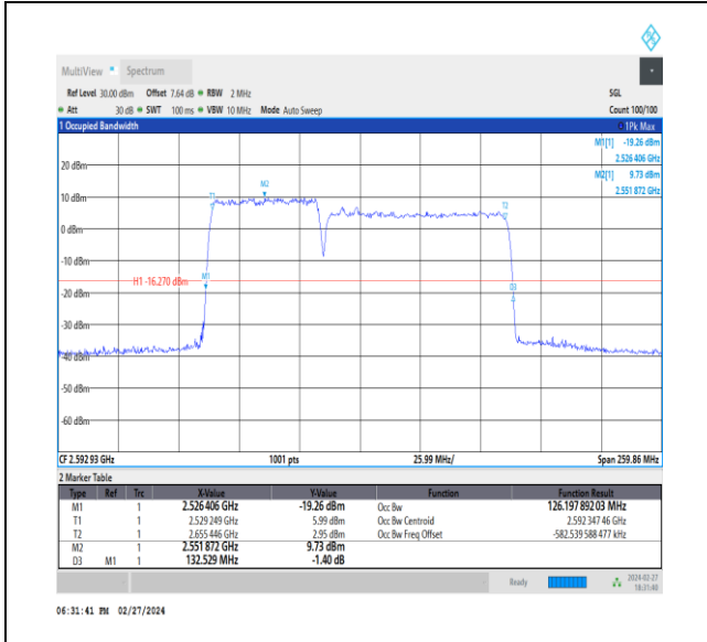
NTVN_CA_n41C_PC3_30+30_50+80_M+M_Ant1_TID6_1_#1
