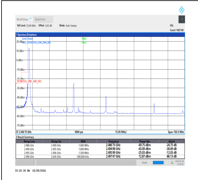
NTNV_CA_n41C_PC3_30+30_40+100_L+L_TID1_1_#1
