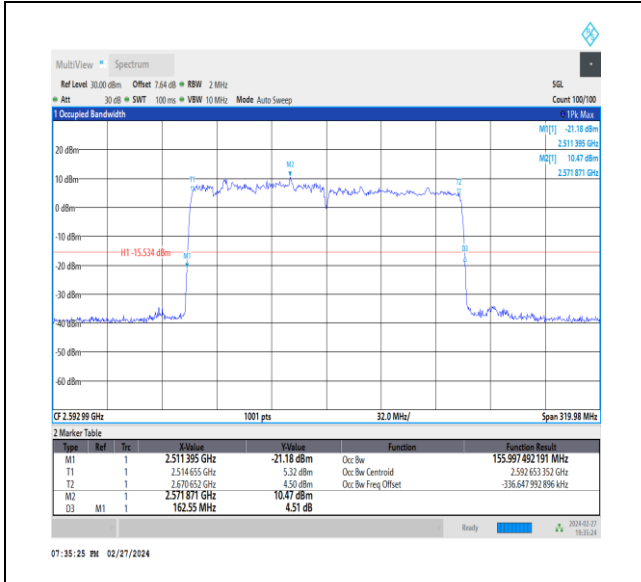
NTNV_CA_n41C_PC3_30+30_80+80_M+M_Ant1_TID7_1_#1
