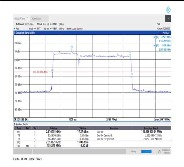
NTVN_CA_n41C_PC3_30+30_50+100_M+M_Ant1_TID6_1_#1
