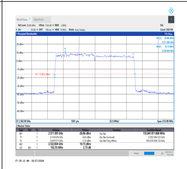
NTVN_CA_n41C_PC3_30+30_80+80_M+M_Ant1_TID6_1_#1
