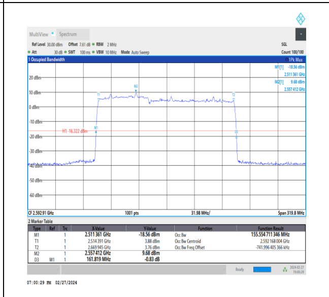
NTVN_CA_n41C_PC3_30+30_60+100_M+M_Ant1_TID5_1_#1
