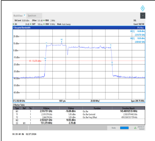
NTVN_CA_n41C_PC3_30+30_50+100_M+M_Ant1_TID1_1_#1
