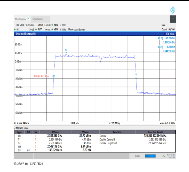
NTVN_CA_n41C_PC3_30+30_80+60_M+M_Ant1_TID2_1_#1
