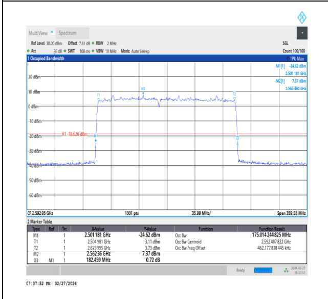
NTVN_CA_n41C_PC3_30+30_80+100_M+M_Ant1_TID2_1_#1
