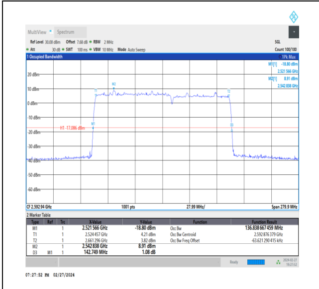
NTNV_CA_n41C_PC3_30+30_80+60_M+M_Ant1_TID5_1_#1
