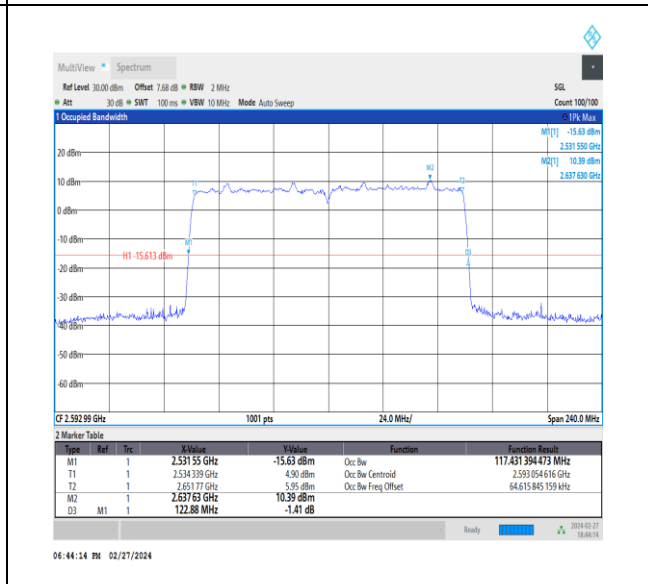
NTVN_CA_n41C_PC3_30+30_60+60_M+M_Ant1_TID3_1_#1
