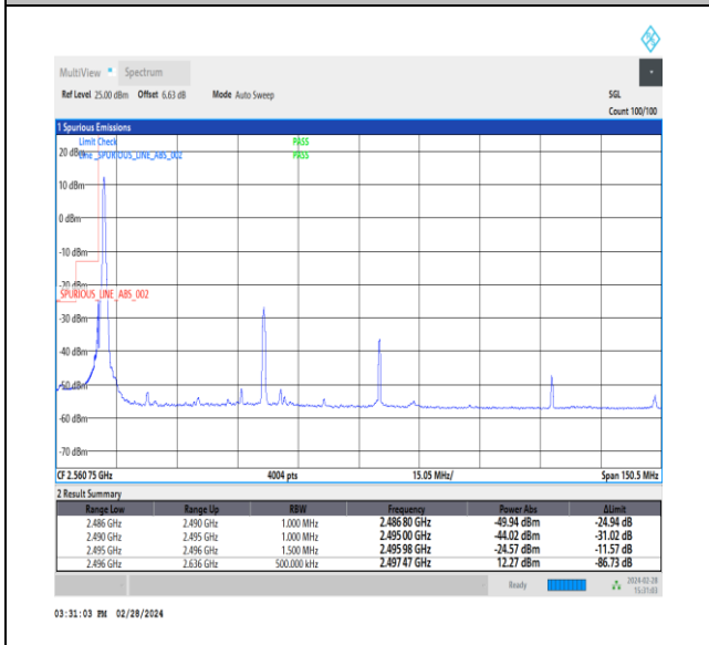
NTNV_CA_n41C_PC3_30+30_40+100_L+L_TID4_1_#1
