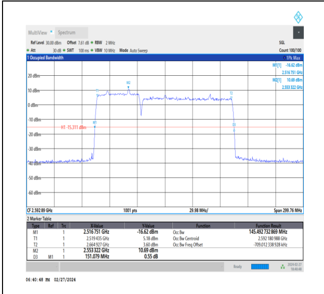
NTVN_CA_n41C_PC3_30+30_50+100_M+M_Ant1_TID5_1_#1
