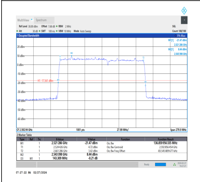
NTVN_CA_n41C_PC3_30+30_80+60_M+M_Ant1_TID3_1_#1
