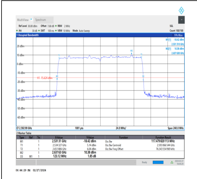
NTVN_CA_n41C_PC3_30+30_60+60_M+M_Ant1_TID4_1_#1
