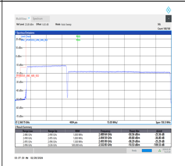
NTNV_CA_n41C_PC3_30+30_40+100_L+L_TID6_1_#1
