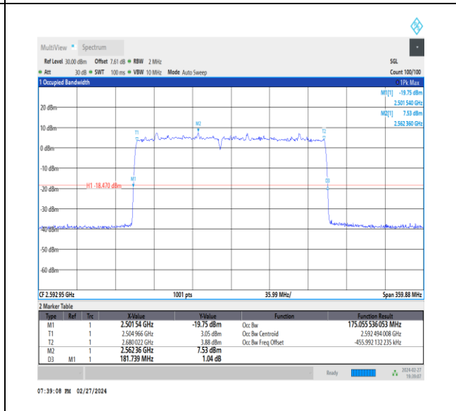
NTVN_CA_n41C_PC3_30+30_80+100_M+M_Ant1_TID7_1_#1
