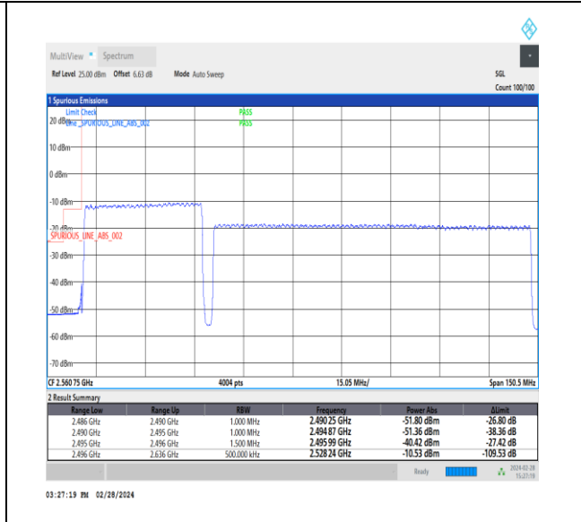
NTNV_CA_n41C_PC3_30+30_40+100_L+L_TID3_1_#1
