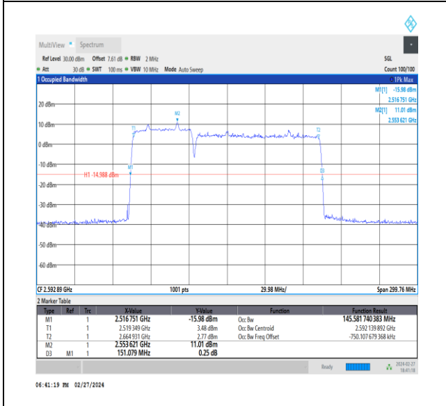
NTVN_CA_n41C_PC3_30+30_50+100_M+M_Ant1_TID7_1_#1
