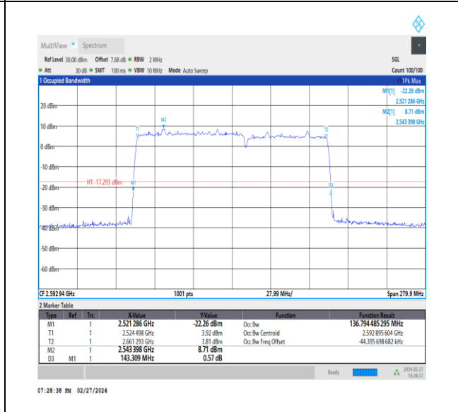
NTNV_CA_n41C_PC3_30+30_80+60_M+M_Ant1_TID8_1_#1
