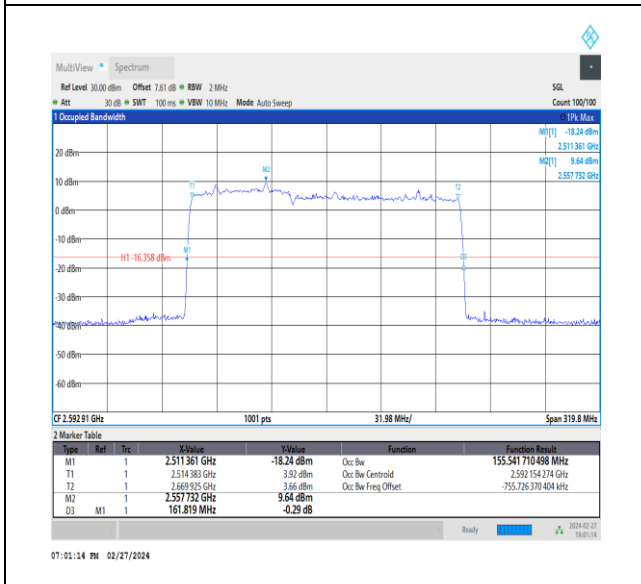
NTNV_CA_n41C_PC3_30+30_60+100_M+M_Ant1_TID8 _1_#1
