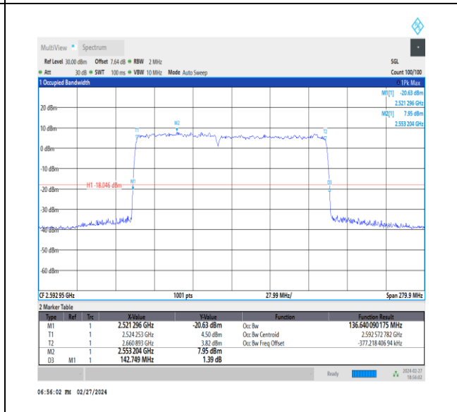
NTNV_CA_n41C_PC3_30+30_60+80_M+M_Ant1_TID2_1_#1
