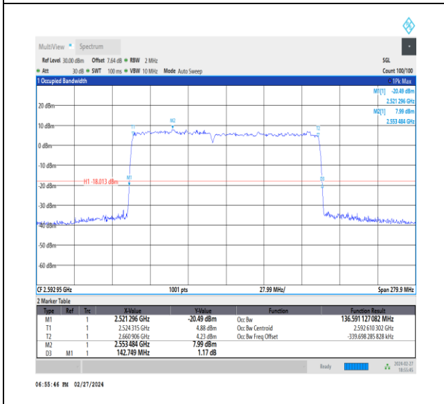
NTNV_CA_n41C_PC3_30+30_60+80_M+M_Ant1_TID1_1_#1
