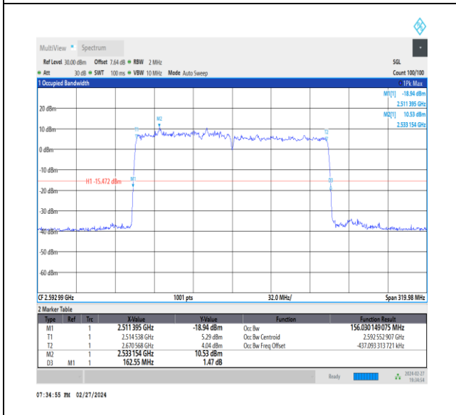
NTVN_CA_n41C_PC3_30+30_80+80_M+M_Ant1_TID5_1_#1
