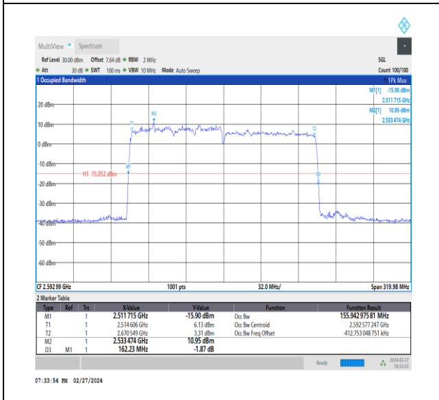
NTNV_CA_n41C_PC3_30+30_80+80_M+M_Ant1_TID1_1_#1
