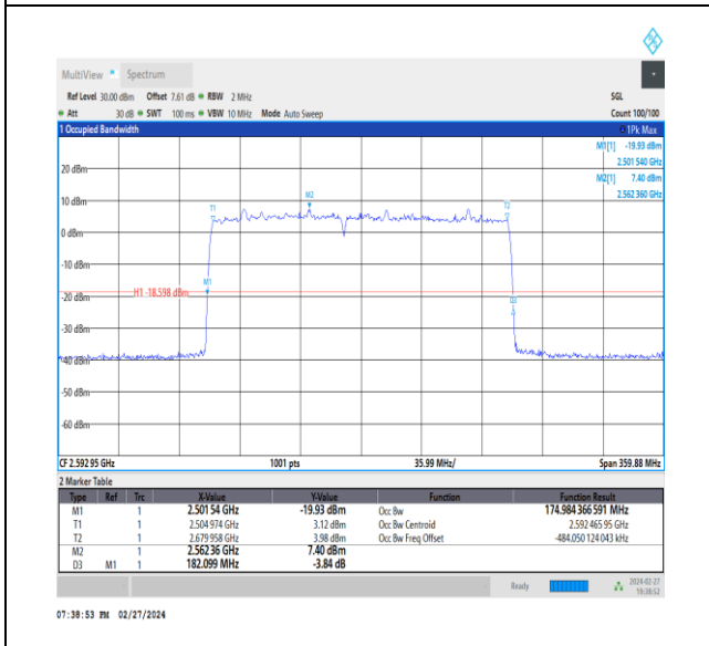
NTVN_CA_n41C_PC3_30+30_80+100_M+M_Ant1_TID6_1_#1
