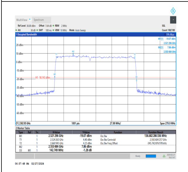
NTNV_CA_n41C_PC3_30+30_60+80_M+M_Ant1_TID9_1_#1
