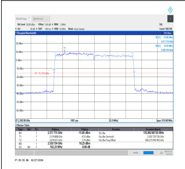
NTNV_CA_n41C_PC3_30+30_80+80_M+M_Ant1_TID9_1_#1
