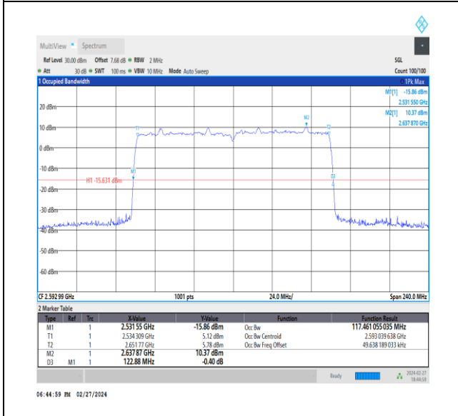
NTVN_CA_n41C_PC3_30+30_60+60_M+M_Ant1_TID6_1_#1
