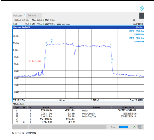
NTVN_CA_n41C_PC3_30+30_50+60_M+M_Ant1_TID3_1_#1
