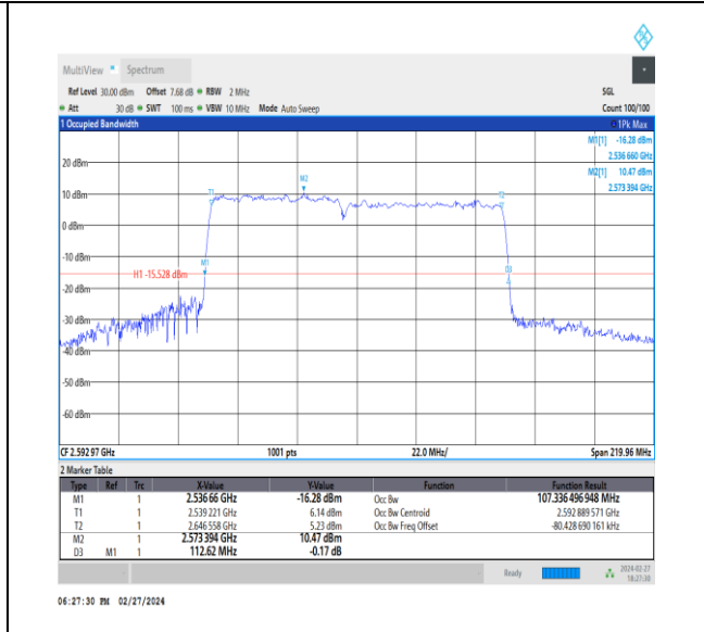
NTVN_CA_n41C_PC3_30+30_50+60_M+M_Ant1_TID8_1_#1
