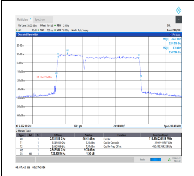
NTVN_CA_n41C_PC3_30+30_40+80_M+M_Ant1_TID9_1_#1
