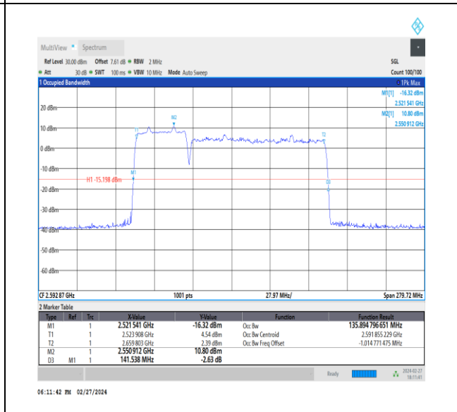
NTVN_CA_n41C_PC3_30+30_40+100_M+M_Ant1_TID7_1_#1
