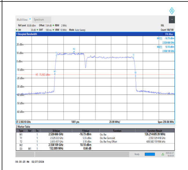
NTVN_CA_n41C_PC3_30+30_50+80_M+M_Ant1_TID1_1_#1
