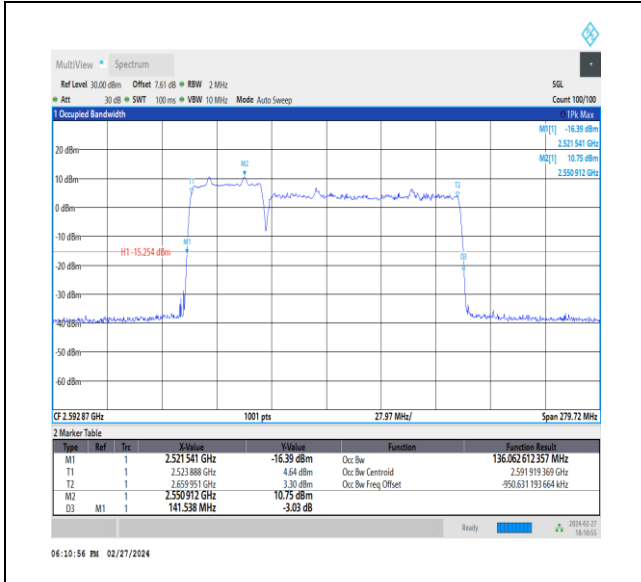
NTVN_CA_n41C_PC3_30+30_40+100_M+M_Ant1_TID4_1_#1
