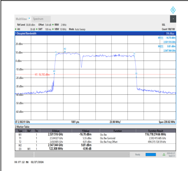
NTVN_CA_n41C_PC3_30+30_40+80_M+M_Ant1_TID7_1_#1
