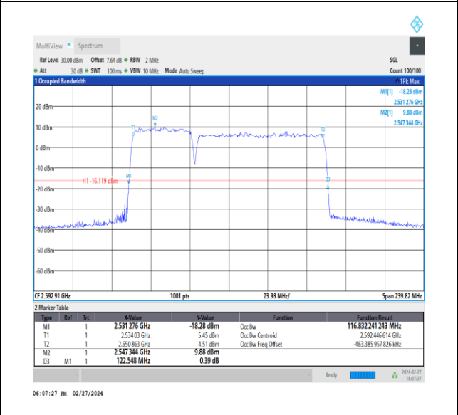
NTVN_CA_n41C_PC3_30+30_40+80_M+M_Ant1_TID8_1_#1
