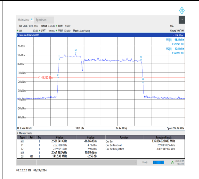
NTVN_CA_n41C_PC3_30+30_40+100_M+M_Ant1_TID9_1_#1
