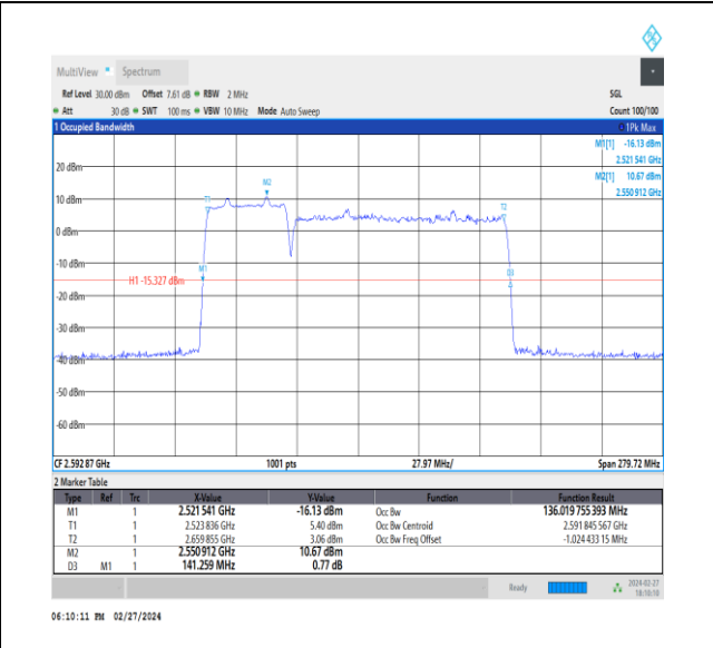
NTVN_CA_n41C_PC3_30+30_40+100_M+M_Ant1_TID1_1_#1
