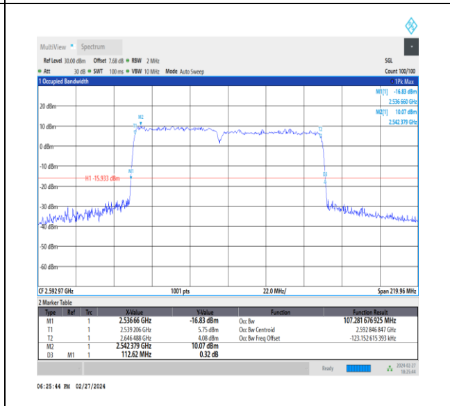
NTVN_CA_n41C_PC3_30+30_50+60_M+M_Ant1_TID6_1_#1
