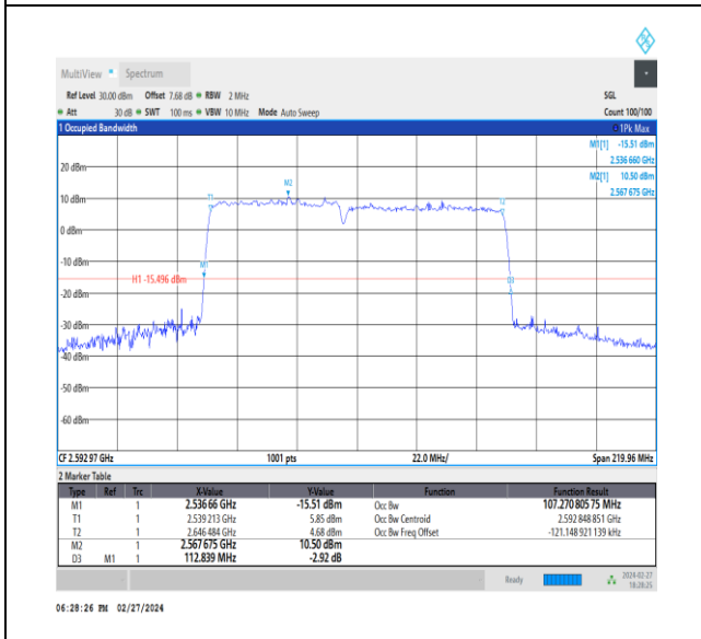
NTVN_CA_n41C_PC3_30+30_50+60_M+M_Ant1_TID9_1_#1
