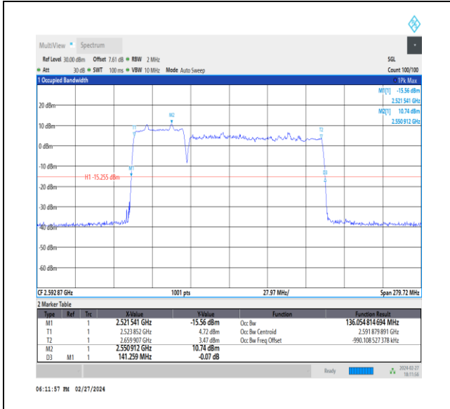
NTVN_CA_n41C_PC3_30+30_40+100_M+M_Ant1_TID8_1_#1
