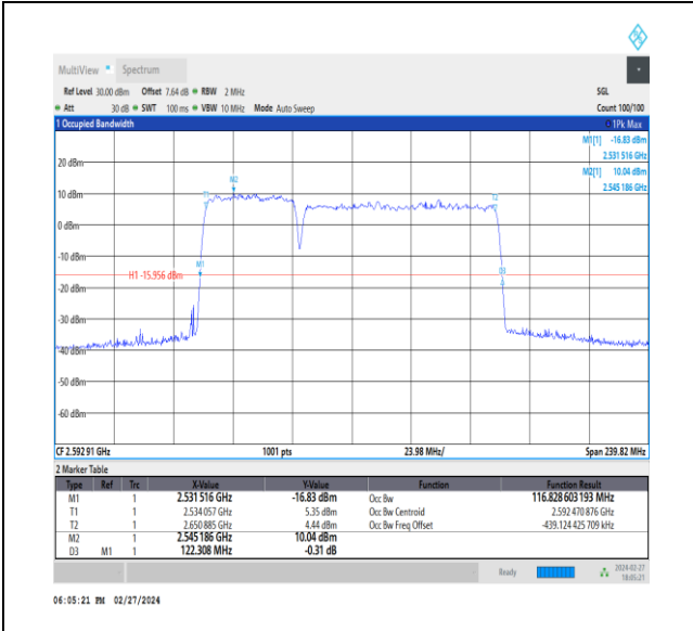
NTVN_CA_n41C_PC3_30+30_40+80_M+M_Ant1_TID5_1_#1
