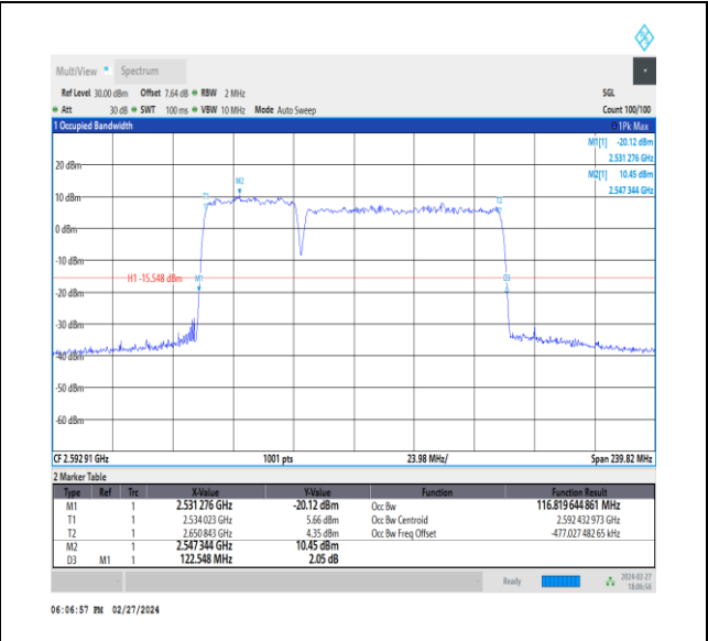
NTVN_CA_n41C_PC3_30+30_40+80_M+M_Ant1_TID6_1_#1
