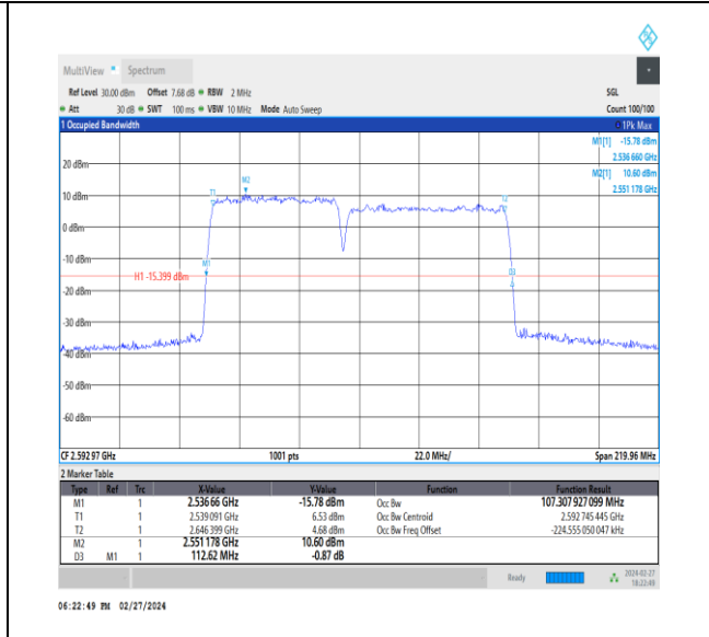
NTVN_CA_n41C_PC3_30+30_50+60_M+M_Ant1_TID4_1_#1
