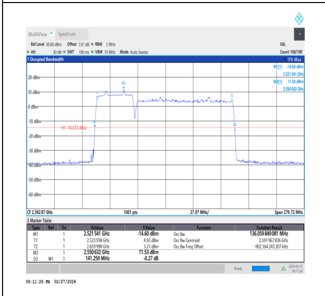
NTVN_CA_n41C_PC3_30+30_40+100_M+M_Ant1_TID6_1_#1
