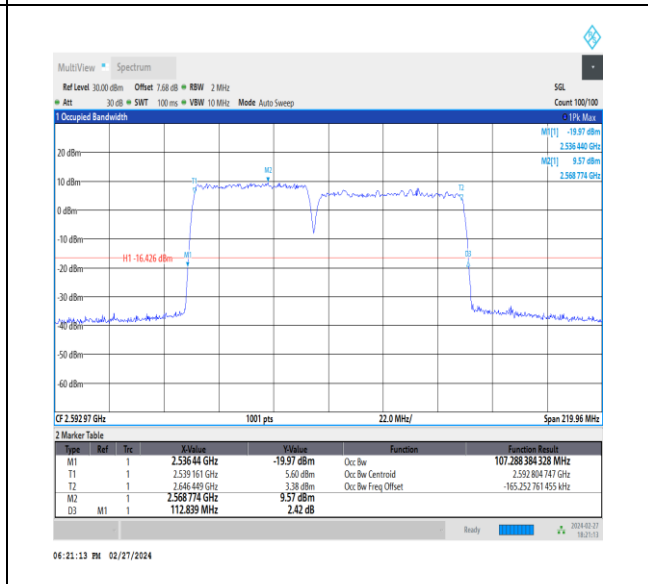
NTVN_CA_n41C_PC3_30+30_50+60_M+M_Ant1_TID2_1_#1
