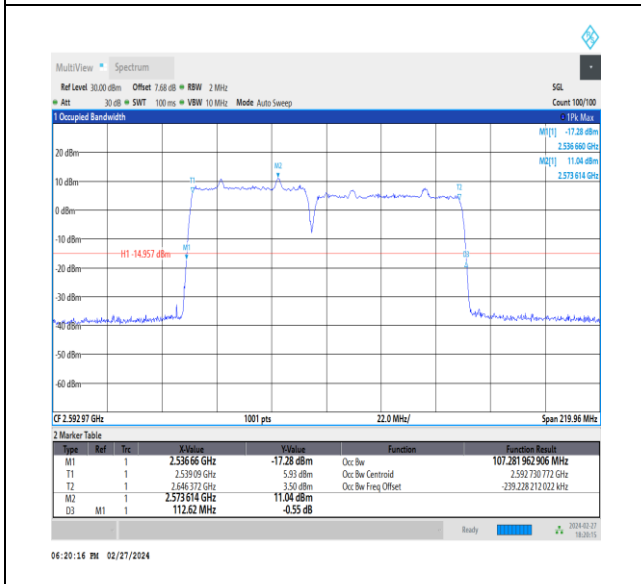
NTVN_CA_n41C_PC3_30+30_50+60_M+M_Ant1_TID1_1_#1
