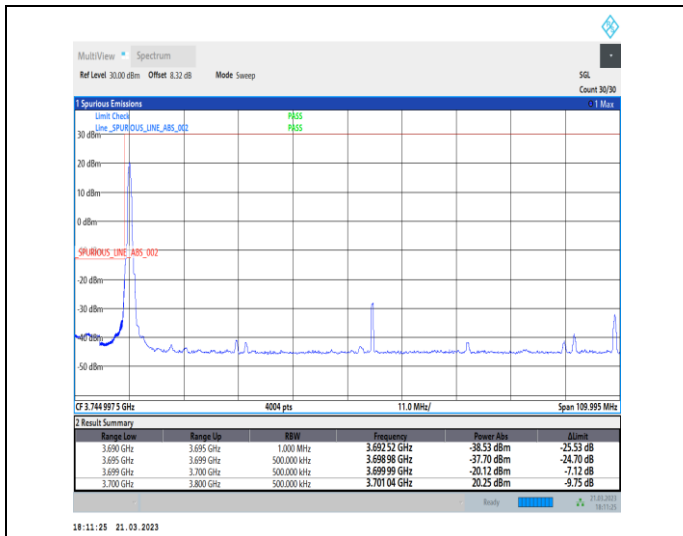
1-N78-3700-3800-30-100-L-4-CP-QPSK-Edge_1RB_L eft-1@0-Ant0-1--PASS-see graph
