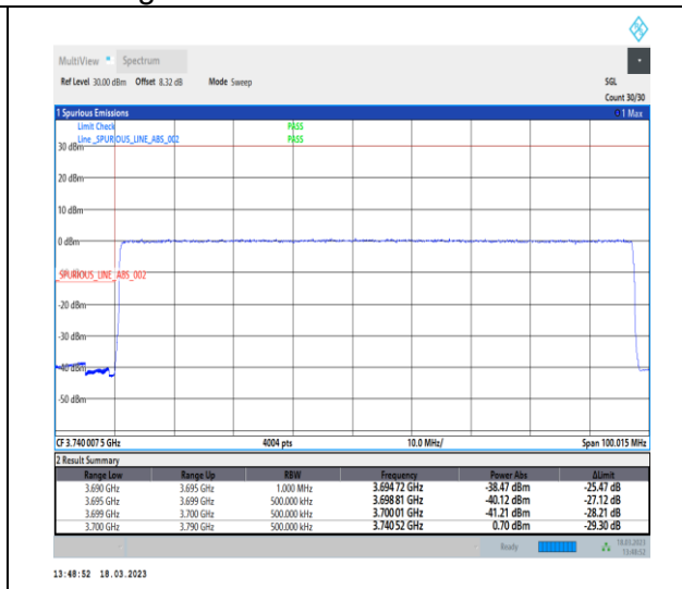
1-N78-3700-3800-30-90-L-3-DFT-PI2BPSK-Outer _Full-240@0-Ant0-1--PASS-see graph
